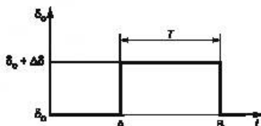
Рисунок 7 — Проверка реакции регулятора угла погасания инвертора на входное ступенчатое воздействие
