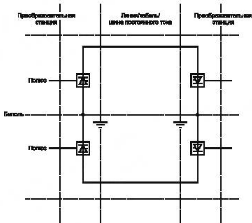
Рисунок 2 — Схема системы ПТВН
