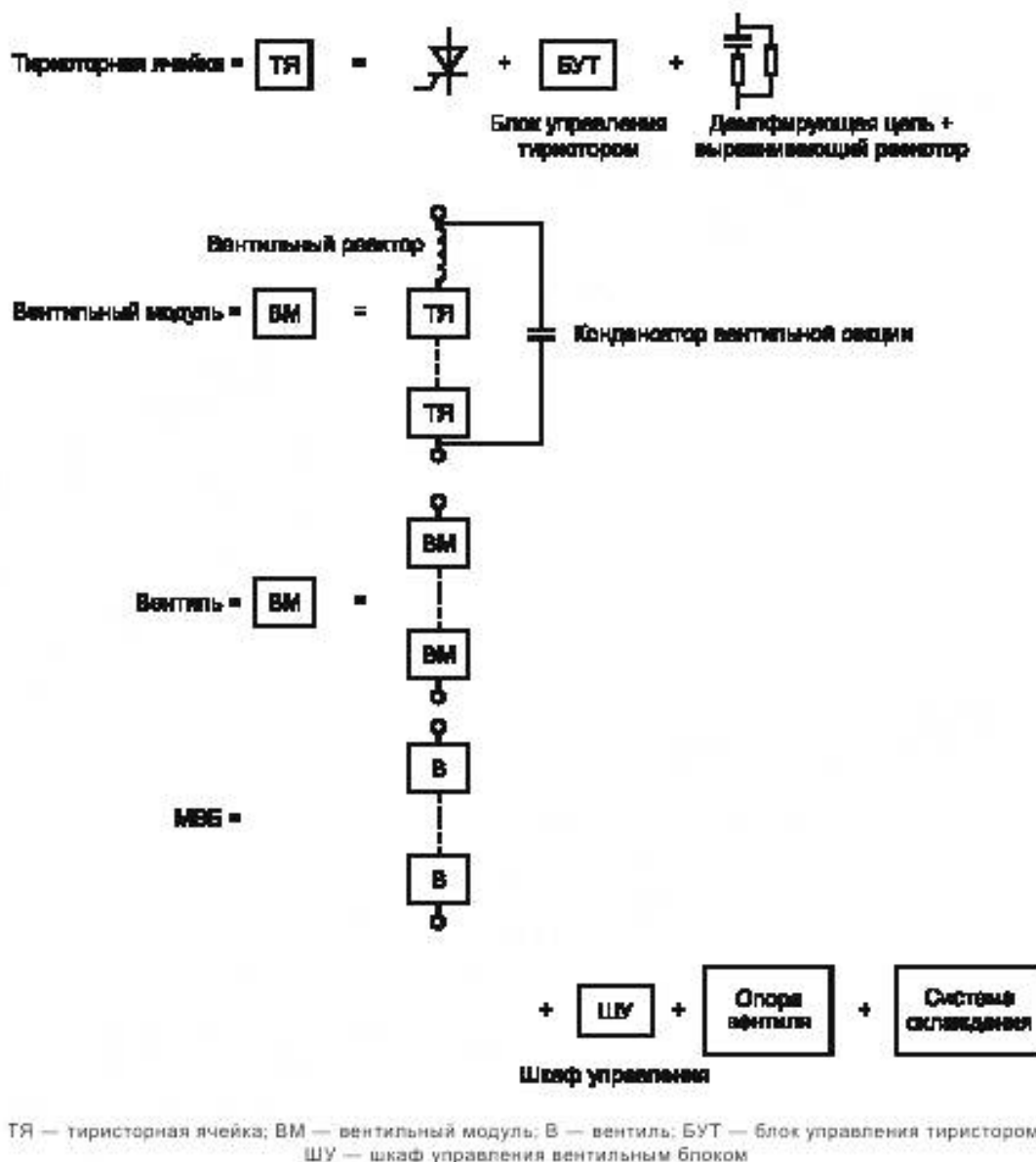
Рисунок 2 — Пример компоновки тиристорного вентиля
