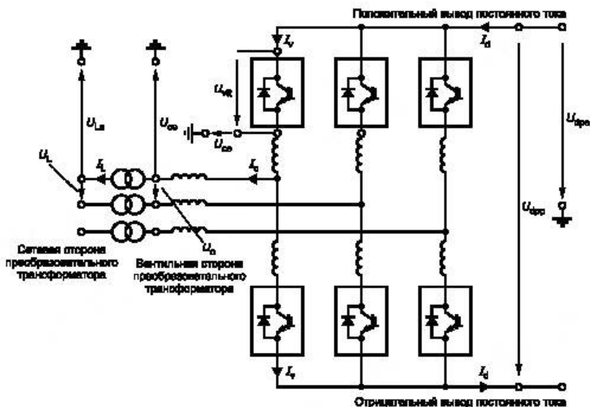
Рисунок 1 — Обозначение электрических величин и терминов, относящихся к преобразователю напряжения
