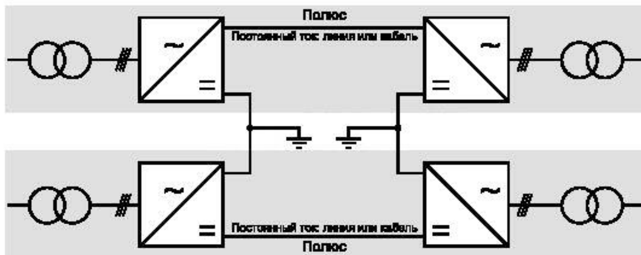
Рисунок 7 — Пример биполярной системы ПТВН с возвратом по земле
