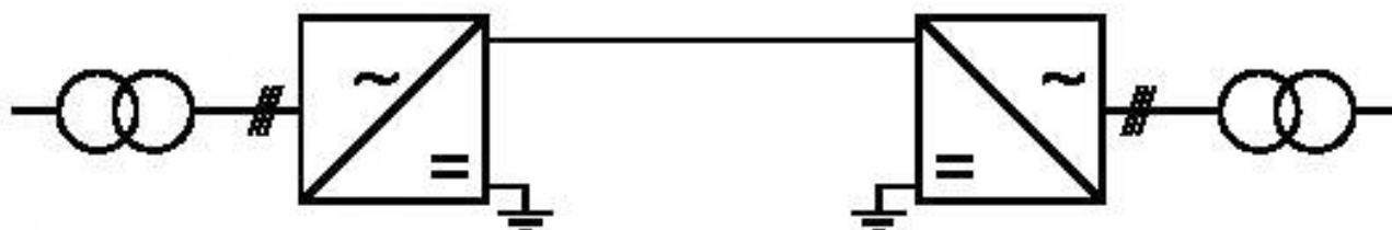
Рисунок 10 — Асимметричная монополярная система ПТВН на основе преобразователей напряжения с возвратом тока по земле
