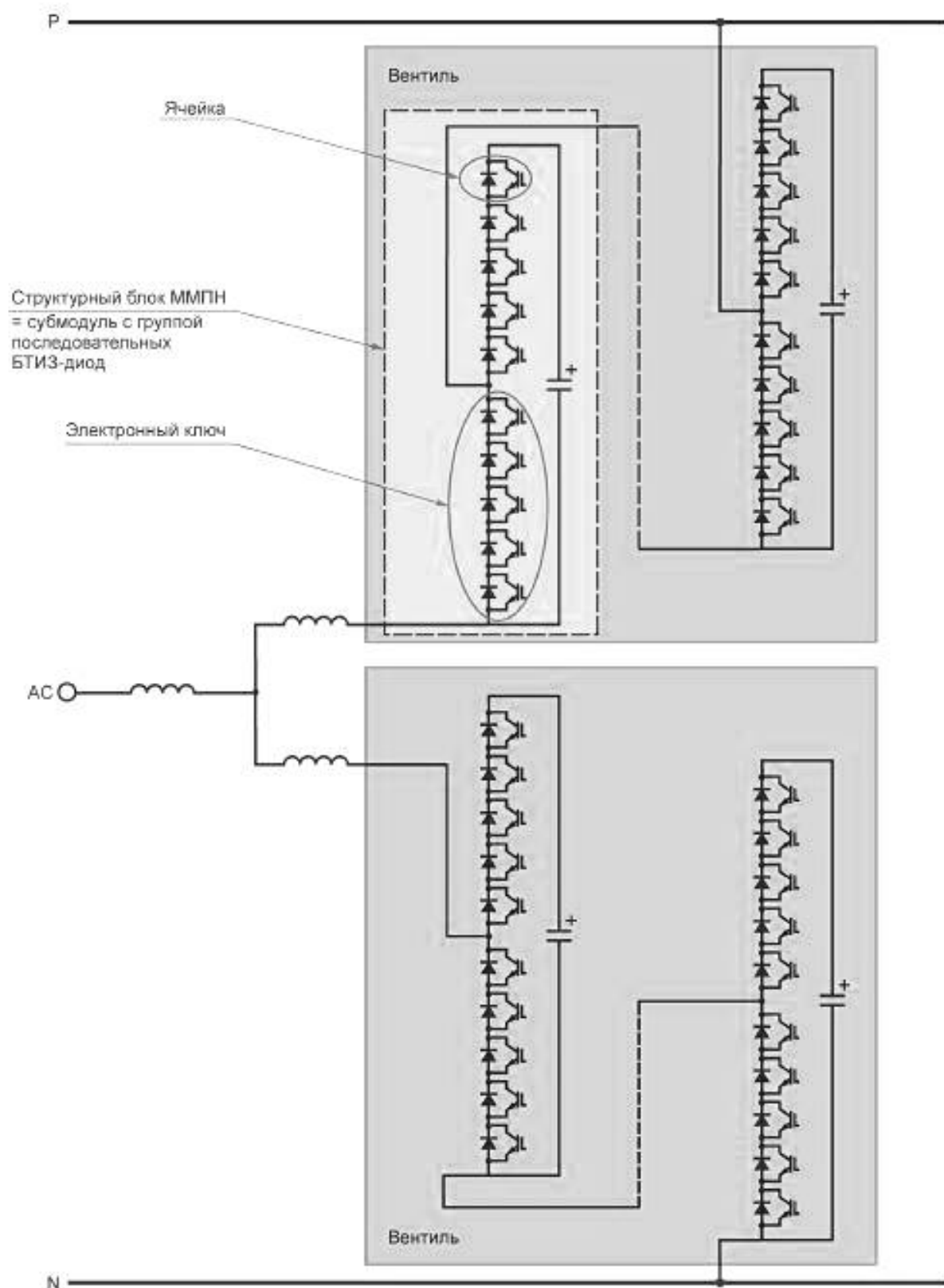
Рисунок 5 — Фазный блок каскадного двухуровневого преобразователя напряжения на основе submodule с группой последовательных ЛПЗ-диод
