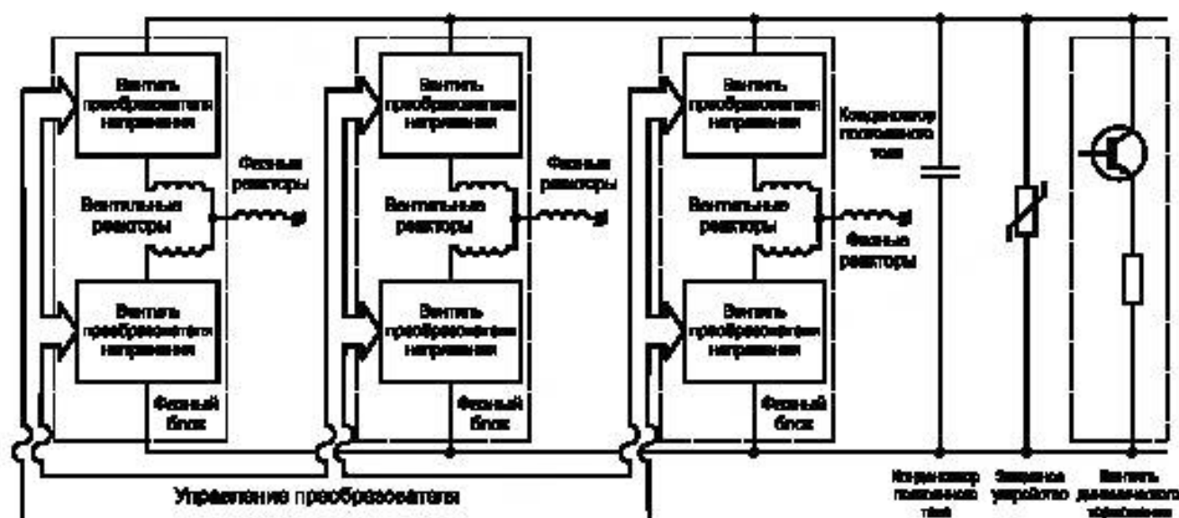
Рисунок 3 — Преобразователь напряжения
