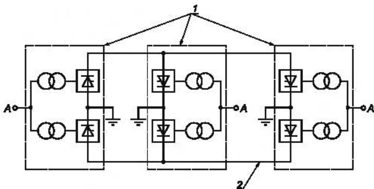
А — система переменного тока; 1 — подстанции ПТВН (см. 8.9); 2 — линия электропередачи ПТВН (см. 8.12)
