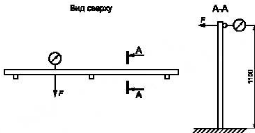
Рисунок 7 — Схема испытания поручней
