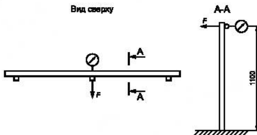
Рисунок 6 — Схема испытания стоек
