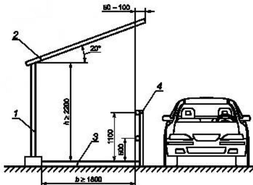
1 — ограждение; 2 — козырек ограждения; 3 — тротуар ограждения; 4 — защитные перила
