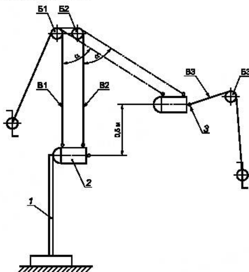
1 — испытательный образец ограждения; 2 — испытательный груз; 3 — расцепное устройство
