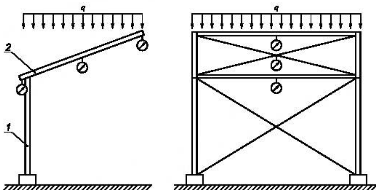
Рисунок 5 — Схема испытания козырька ограждения
