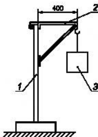
1 — испытательный образец ограждения; 2 — консоль; 3 — контрольный груз
