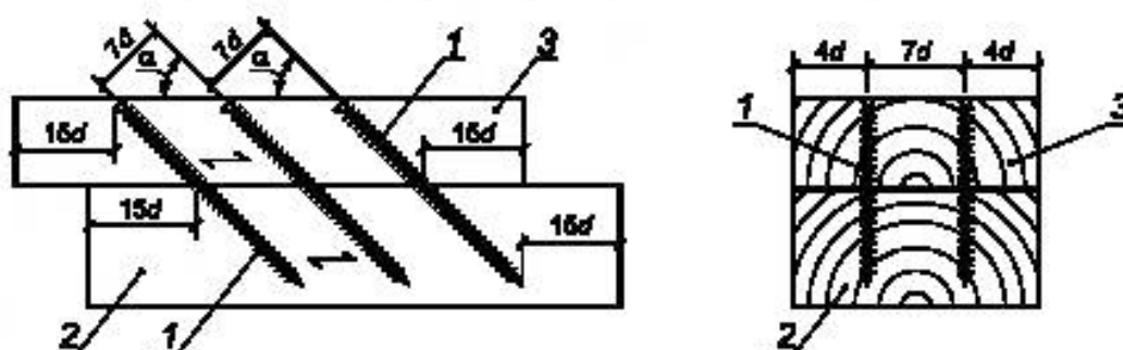
1 — винты; 2 и 3 — элементы соединения из древесины или материалов на ее основе
