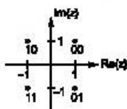
Рисунок 10 — Сигнальное созвездие при модуляции QPSK
