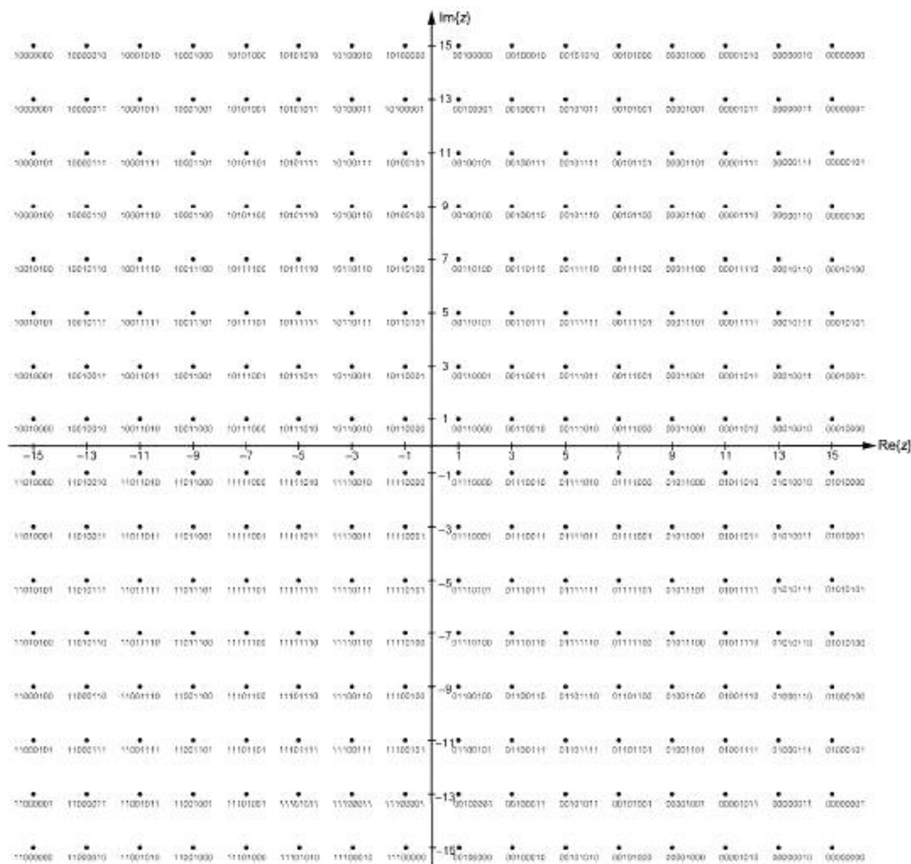
Рисунок 13 — Сигнальное созвездие при модуляции 256-QAM
