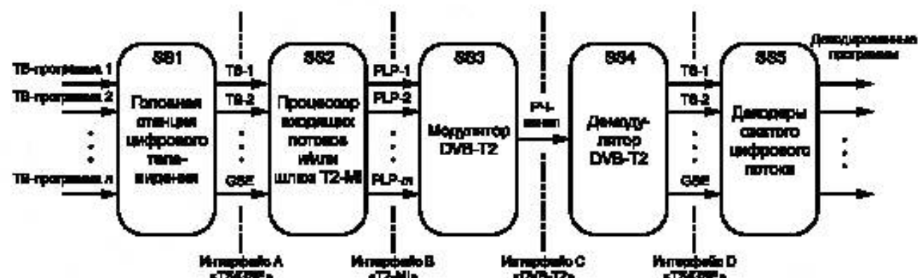
Рисунок 1 — Высокоуровневая архитектура системы DVB-T2
