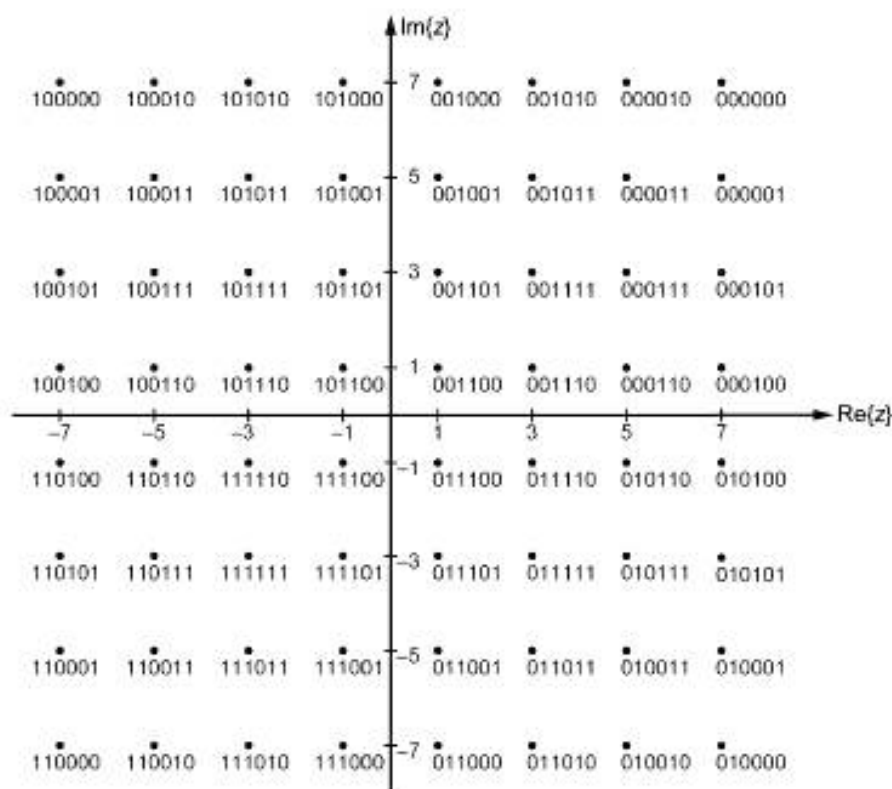
Рисунок 12 — Сигнальное созвездие при модуляции 64-QAM
