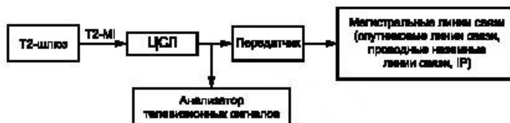
Рисунок 37 — Схема проведения измерений параметров сквозной доставки цифрового телевизионного сигнала по магистральным линиям связи
