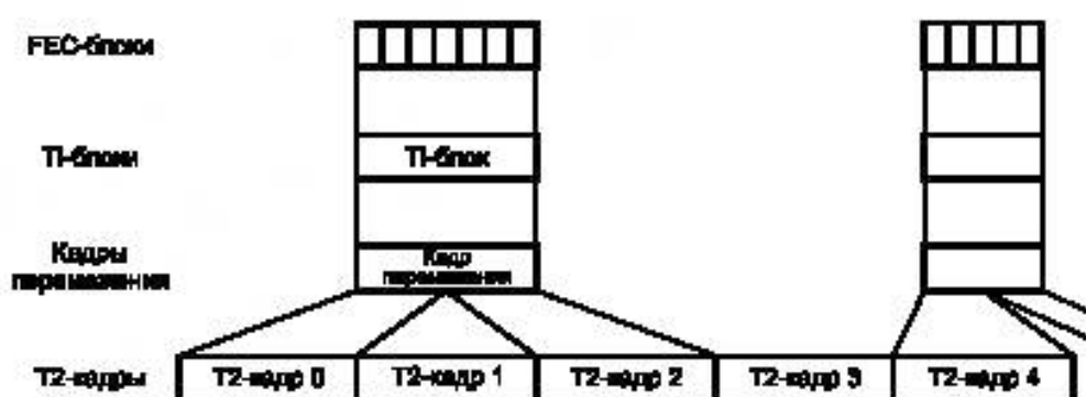
Рисунок 16 — Перемежение по времени для P_1 = 2 , I_{\text{JUMP}} = 2 , N_{T1} = 1
