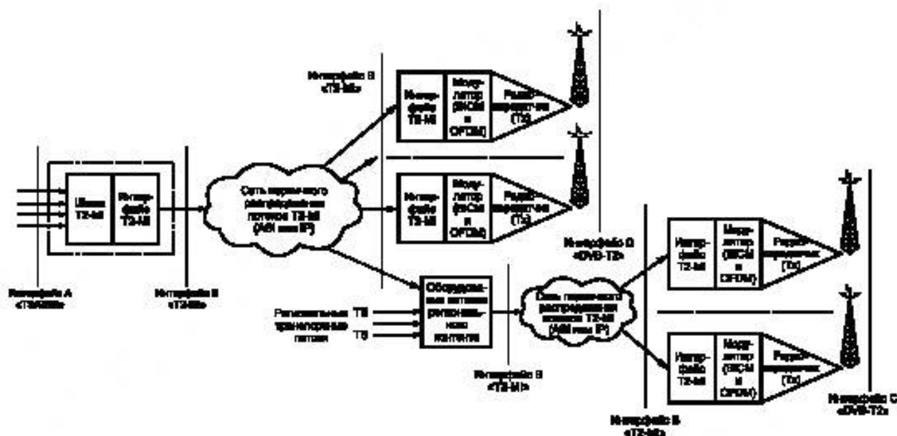
Рисунок 4 — Архитектура передающей части системы DVB-T2, обеспечивающей вставку регионального контента
