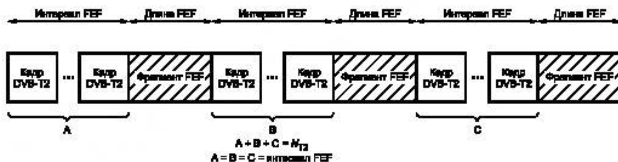
Рисунок 28 — Суперкадр, включающий T2-кадры и фрагменты FEF
