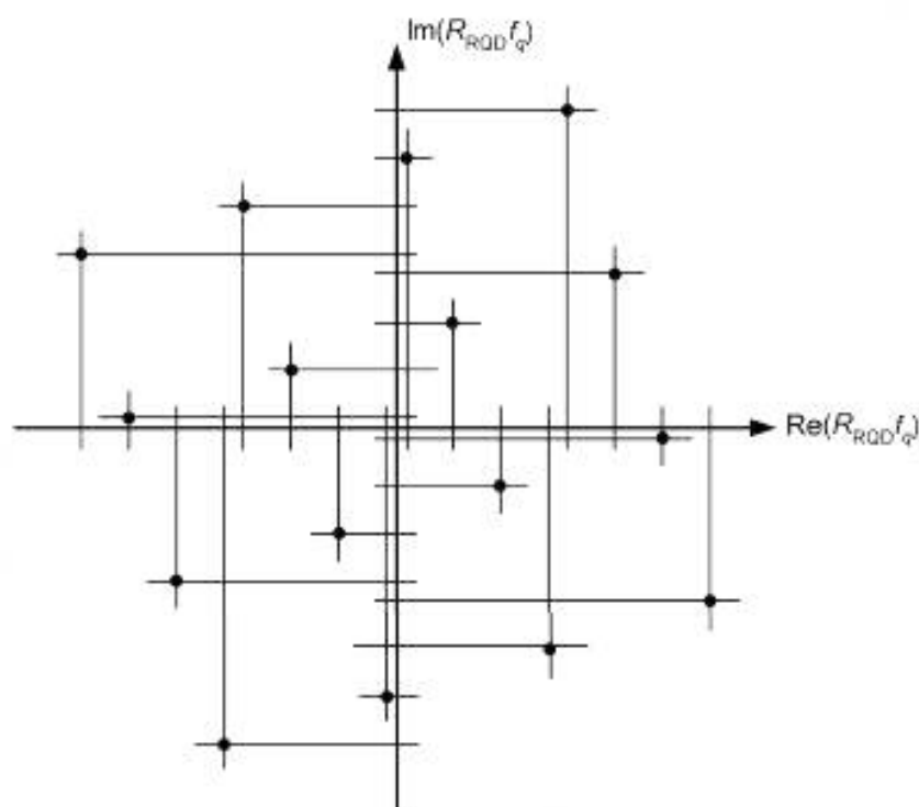
Рисунок 14 — Повернутое созвездие при модуляции 16-QAM
