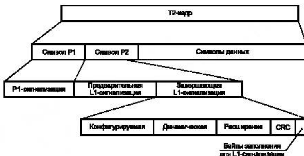
Рисунок 19 — Структура L1-сигнализации
