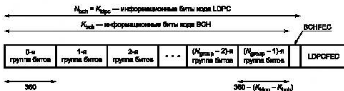
Рисунок 24 — Формат групп битов после LDPC-кодирования данных L1-сигнализации
