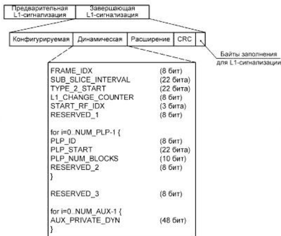
Рисунок 22 — Поля данных динамической завершающей L1-сигнализации
