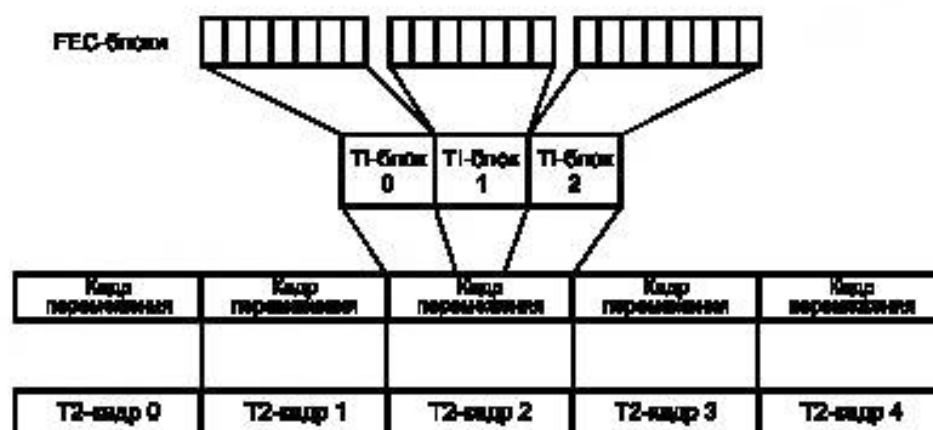
Рисунок 17 — Перемежение по времени для P_1 = 1 , I_{\text{JUMP}} = 1 , N_{T1} = 3
