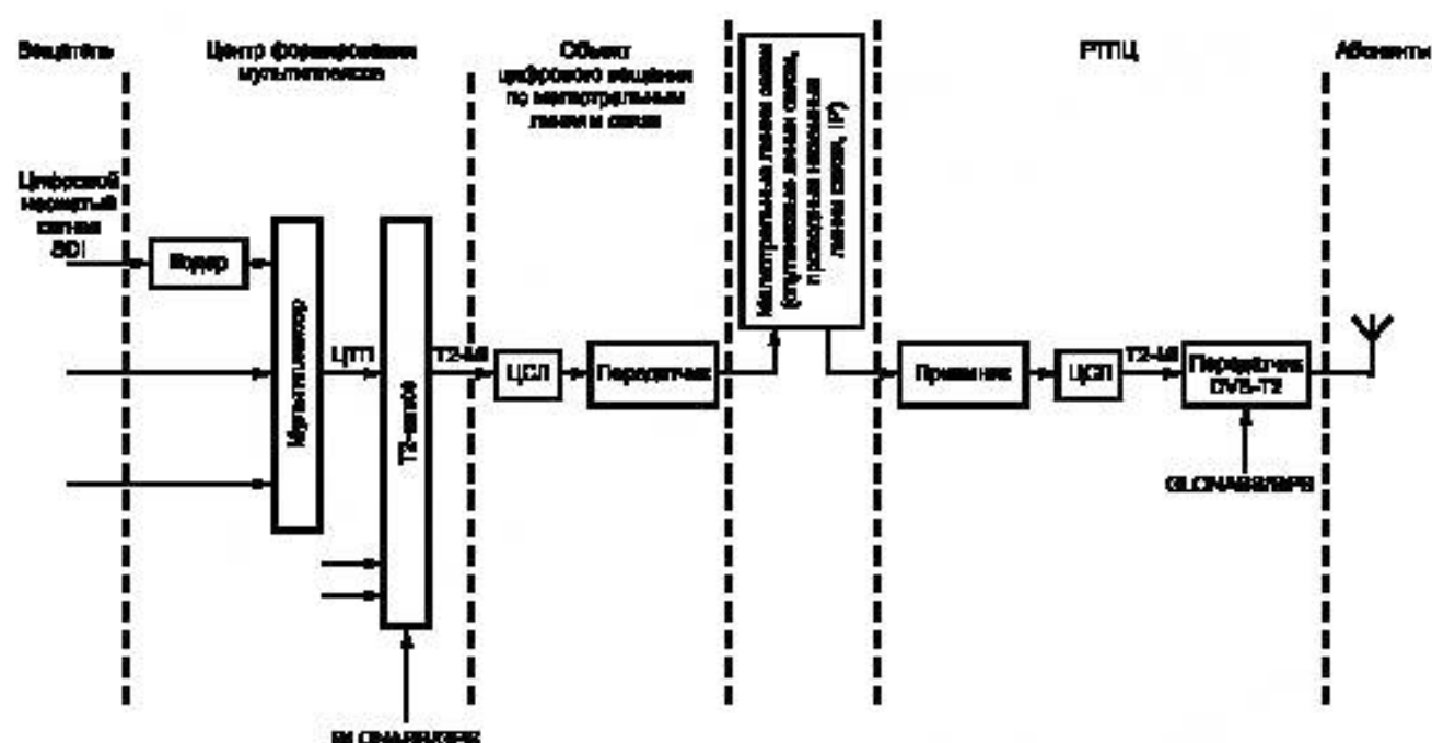
Рисунок 34 — Типовая структурная схема телевизионного вещания
