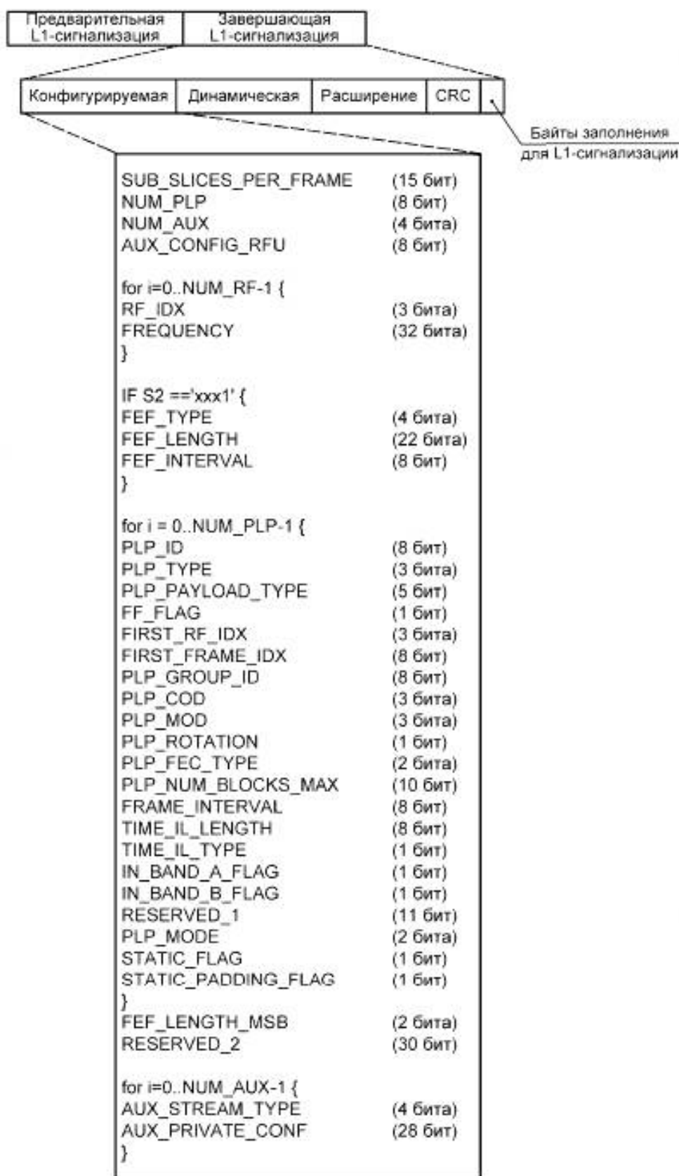
Рисунок 21 — Поля данных конфигурируемой завершающей L1-сигнализации
