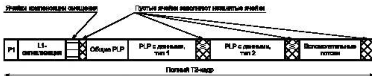
Рисунок 29 — Структура T2-кадра
