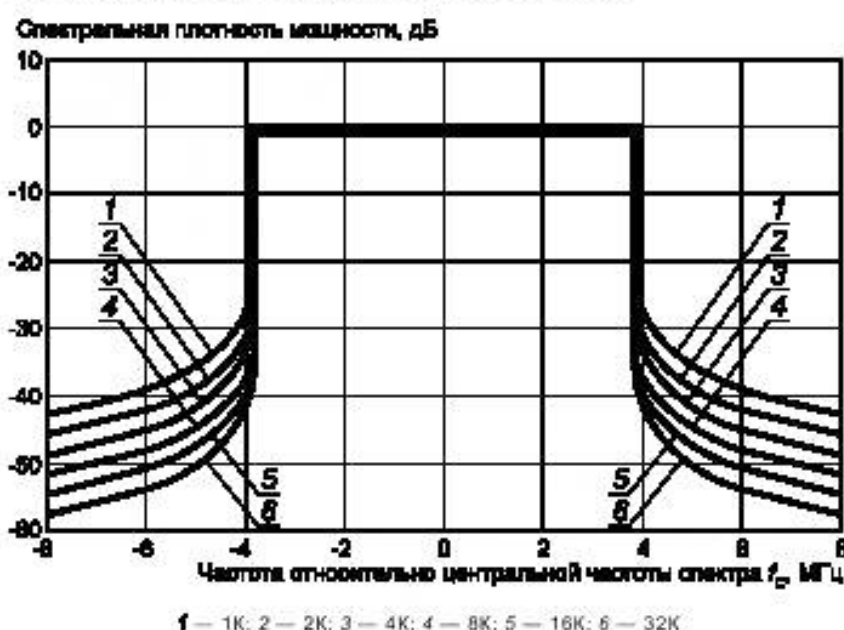
Рисунок 31 — Теоретический спектр сигнала OFDM
