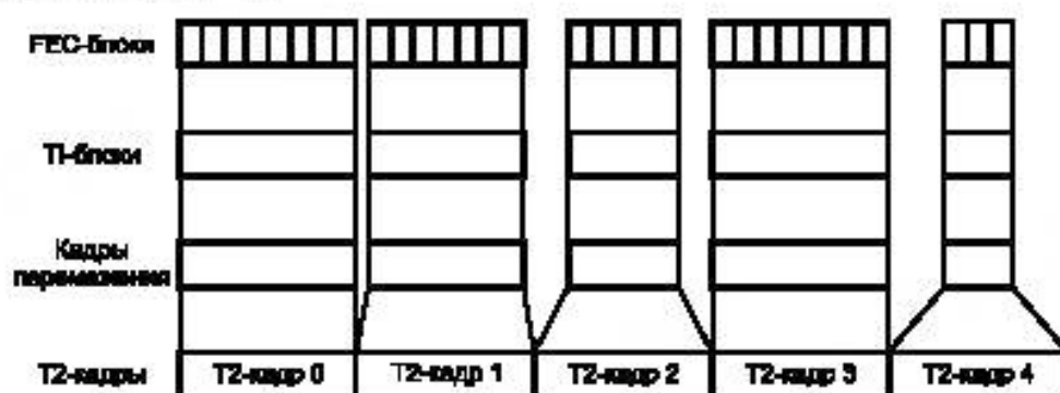
Рисунок 15 — Перемежение по времени для P_1 = 1 , I_{\text{JUMP}} = 1 , N_{T1} = 1
