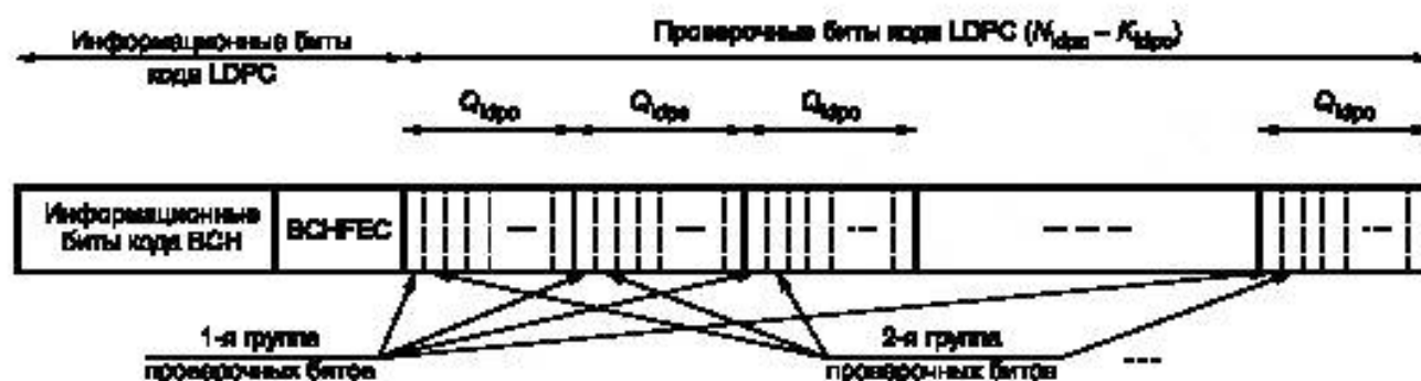
Рисунок 25 — Группы проверочных битов в FEC-блоке
