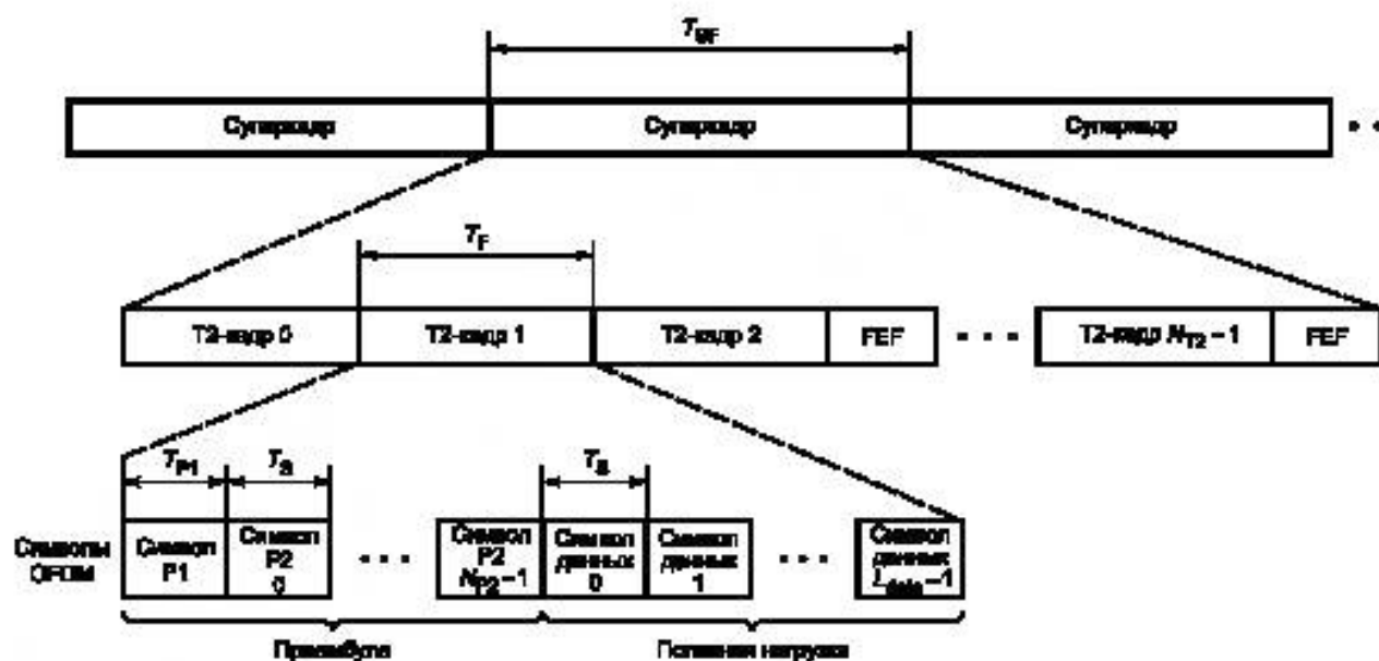
Рисунок 27 — Структура кадров системы DVB-T2 на физическом уровне
