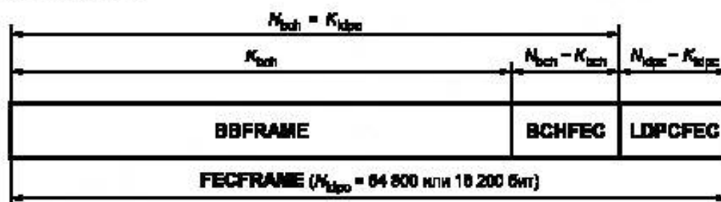
Рисунок 7 — Формат данных перед перемежением по битам
