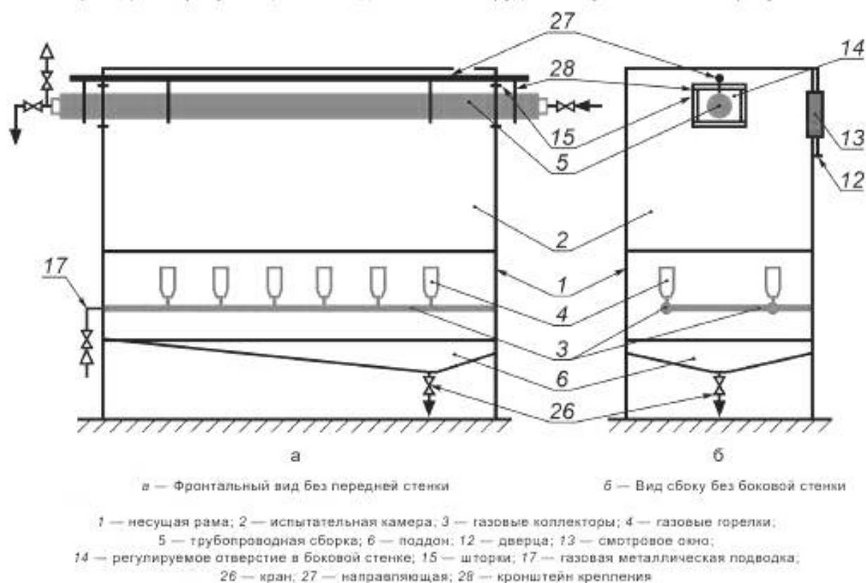
Рисунок 2 — Общий вид установки для испытаний неметаллических трубопроводных сборок
