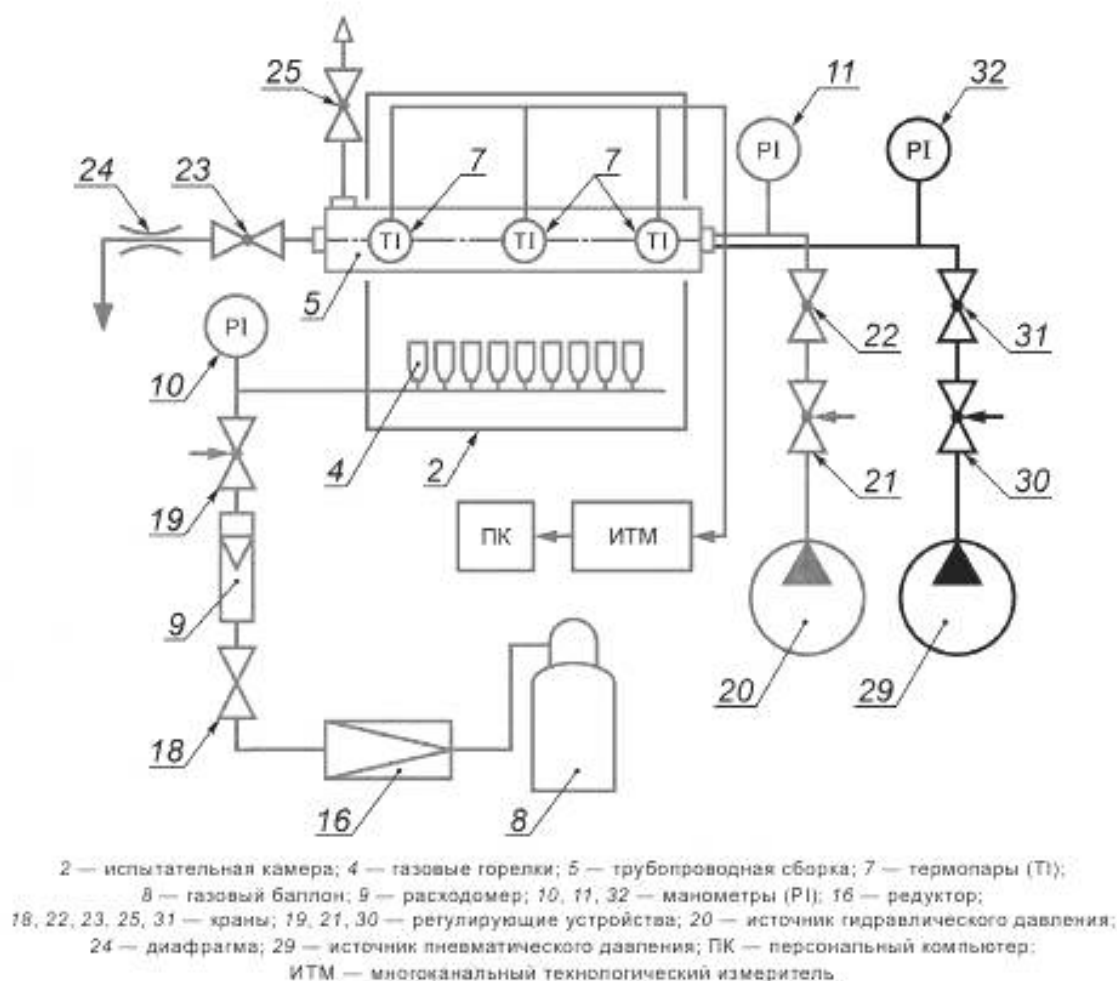
Рисунок 3 — Схема подключения оборудования установки для испытаний неметаллических трубопроводных сборок
