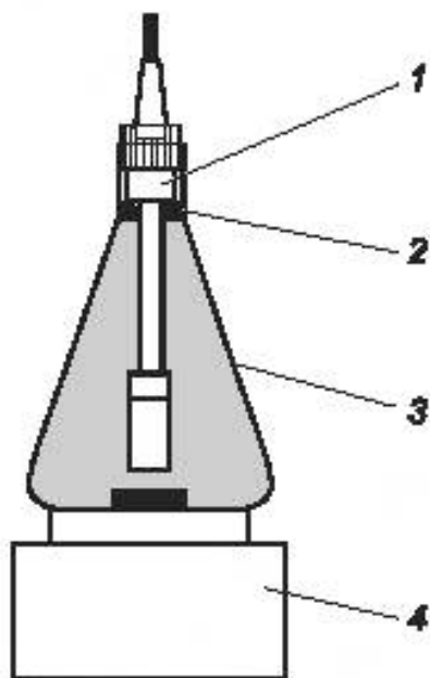
1 — датчик; 2 — резиновое кольцо; 3 — склянка; 4 — магнитная мешалка
