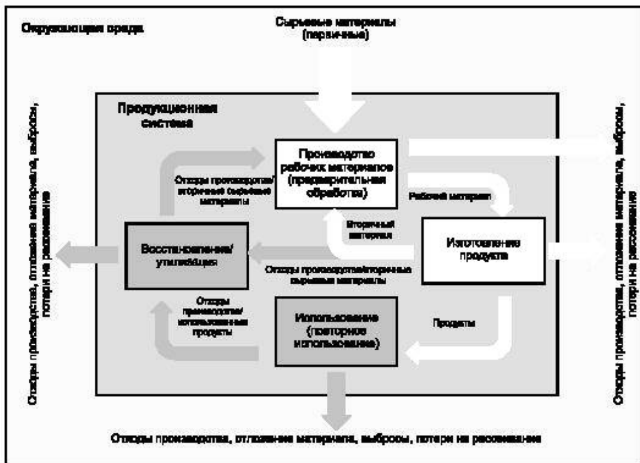
Рисунок 5 — Рассмотрение использования ресурса «от колыбели до ворот». Движение материалов
