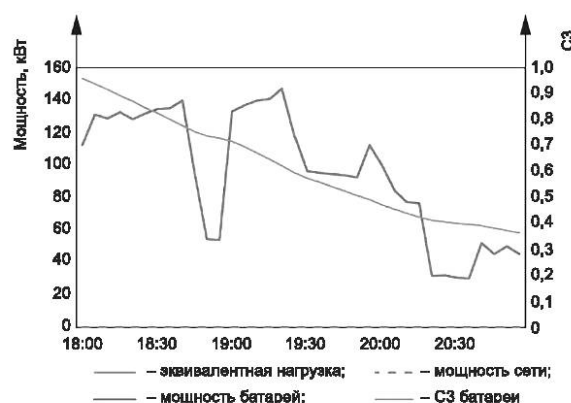
б) Рабочая мощность с 18:00 до 21:00
