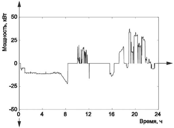
б) Мощность СНЭЭ
