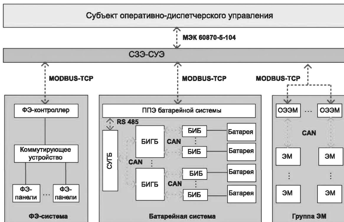
Рисунок 1 — Пример архитектуры коммуникационной системы ЭЗС-ФЭ-СНЭЭ
