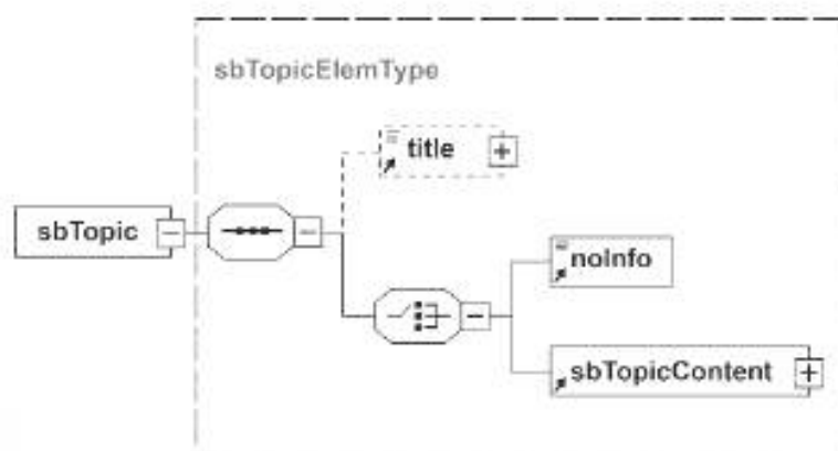
Рисунок 4 — Схема данных элемента «sbTopic»
