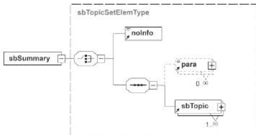
Рисунок 5 — Схема данных элемента «sbSummary»
