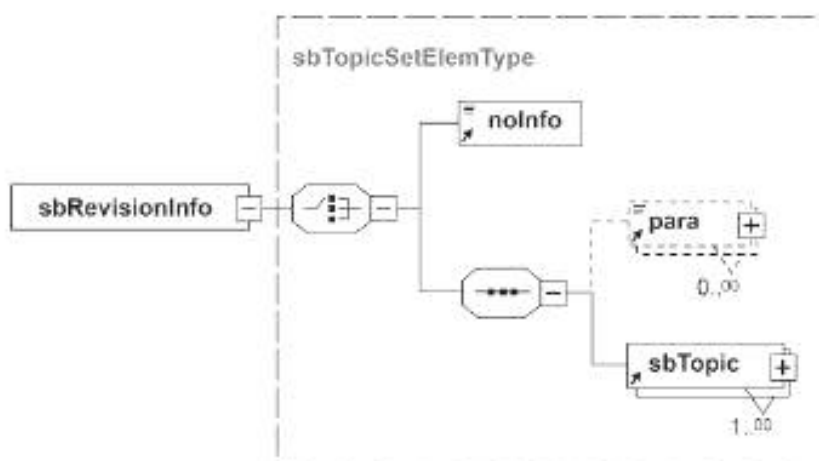
Рисунок 3 — Схема данных элемента «sbRevisionInfo»
