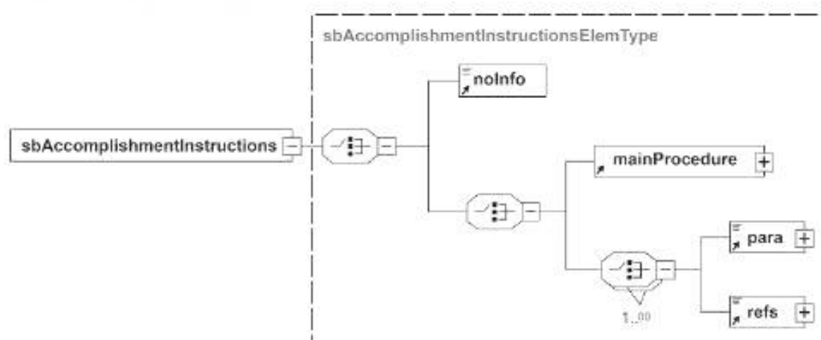
Рисунок 8 — Схема данных элемента «sbAccomplishmentInstructions»
