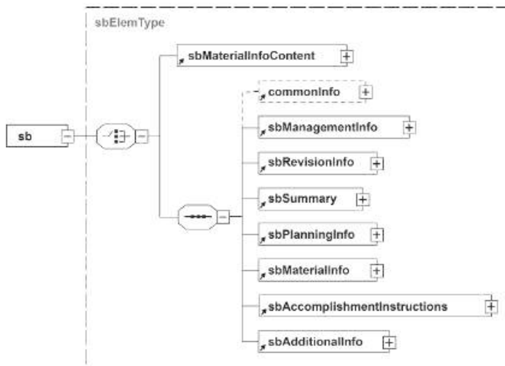
Рисунок 2 — Схема данных элемента «sb»
