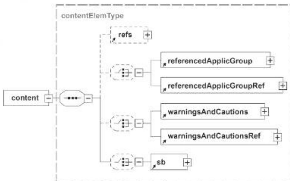
Рисунок 1 — Схема данных элемента «content»
