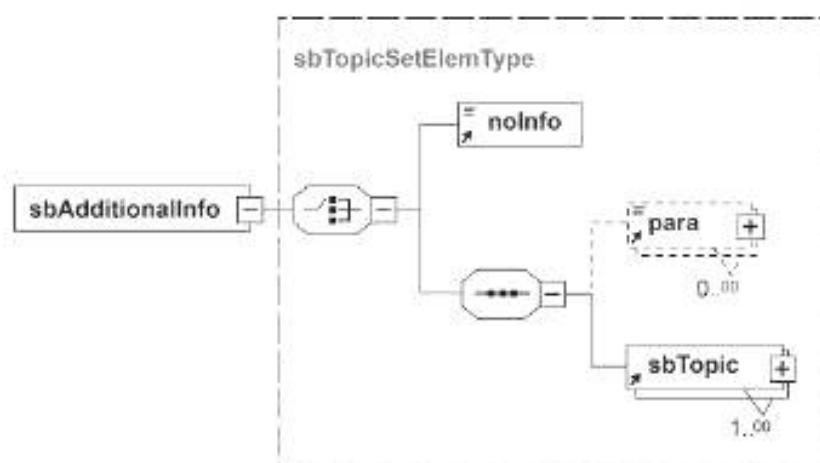
Рисунок 9 — Схема данных элемента «sbAdditionalInfo»
