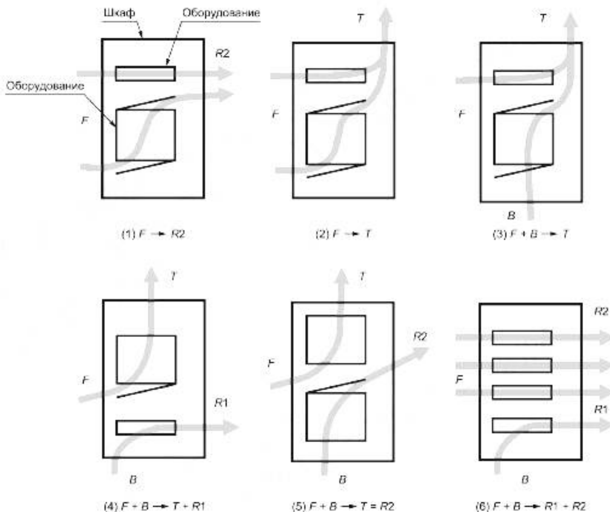
Рисунок 3 — Предпочтительные схемы распределения воздушных потоков
