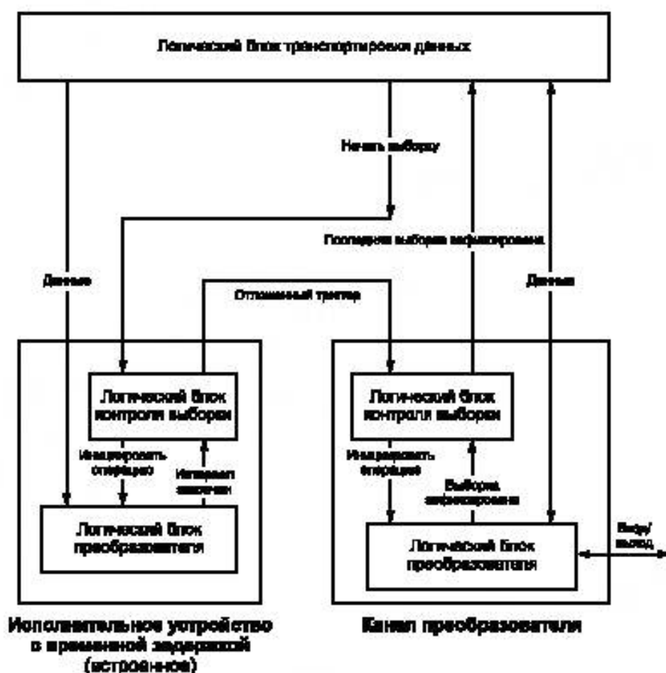
Рисунок М.1 — Канал преобразователя с изменяемым временем задержки триггера
