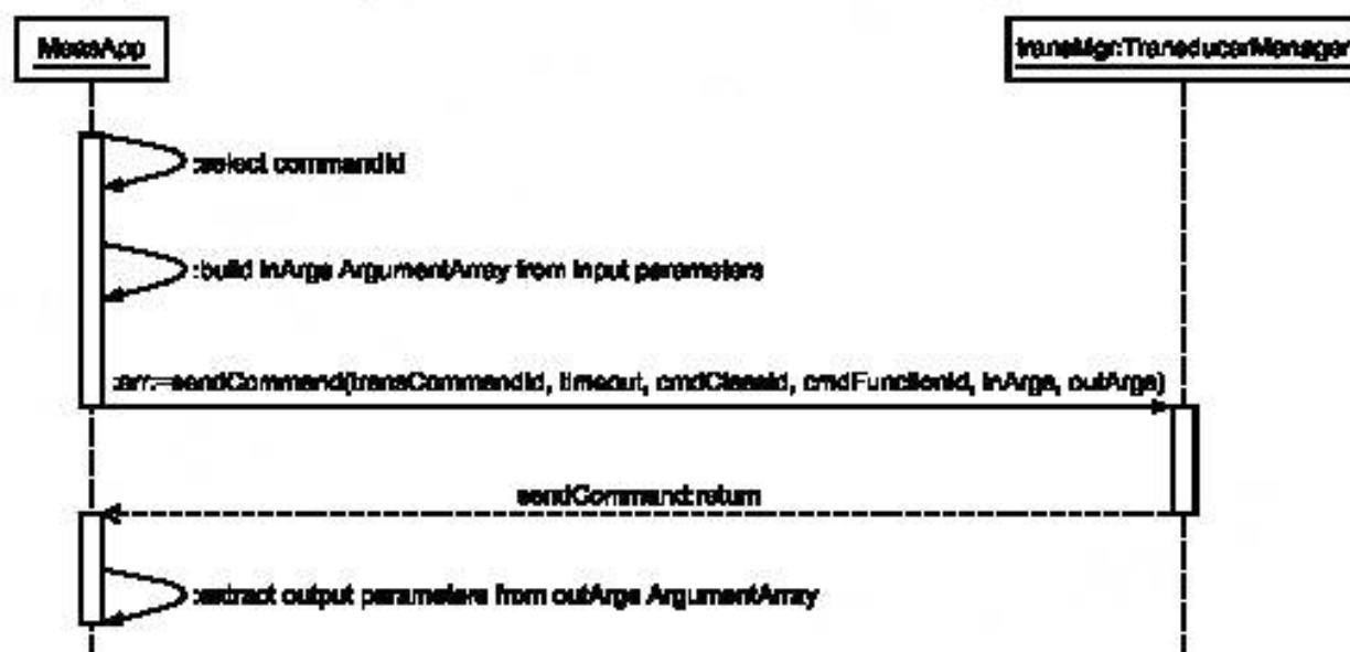
Рисунок В.3 — Диаграмма последовательности действий «SendCommand»
