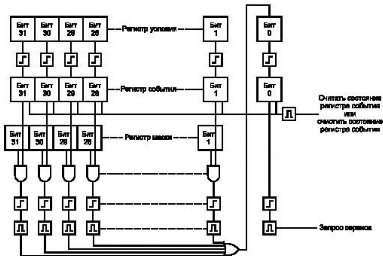
Рисунок 11 — Логика создания сообщений состояния
