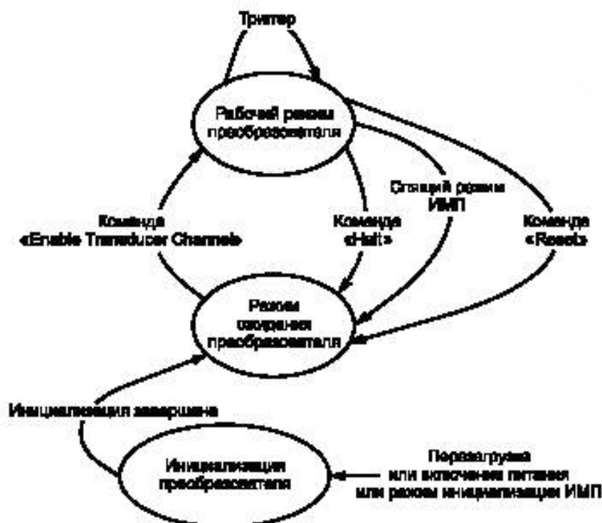
Рисунок 3 — Режимы работы канала преобразователя
