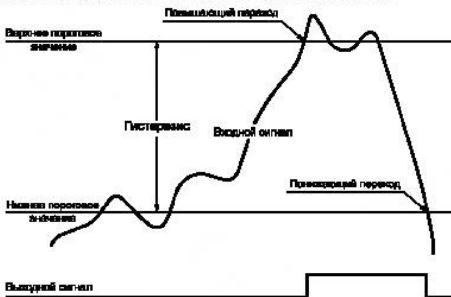
Рисунок 5 — Характеристика аналогового датчика событий
