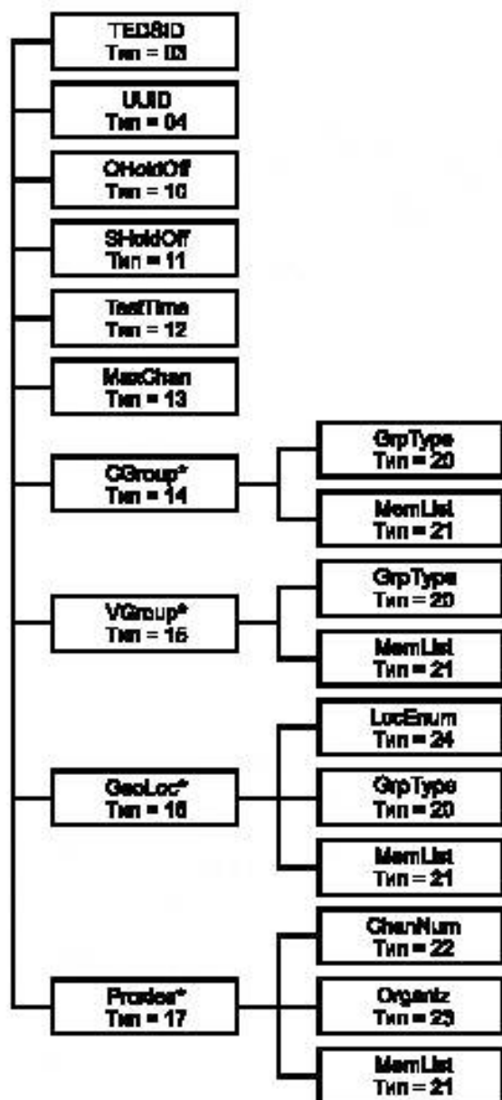
Рисунок 13 — Структура блока данных мета-ЭТДП
