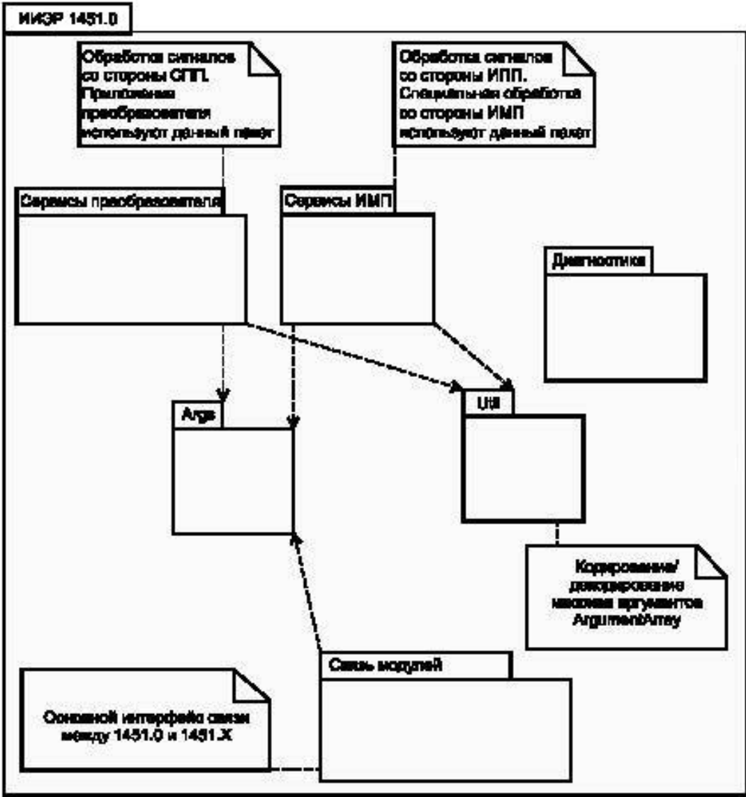
Рисунок 21 — Структура API
