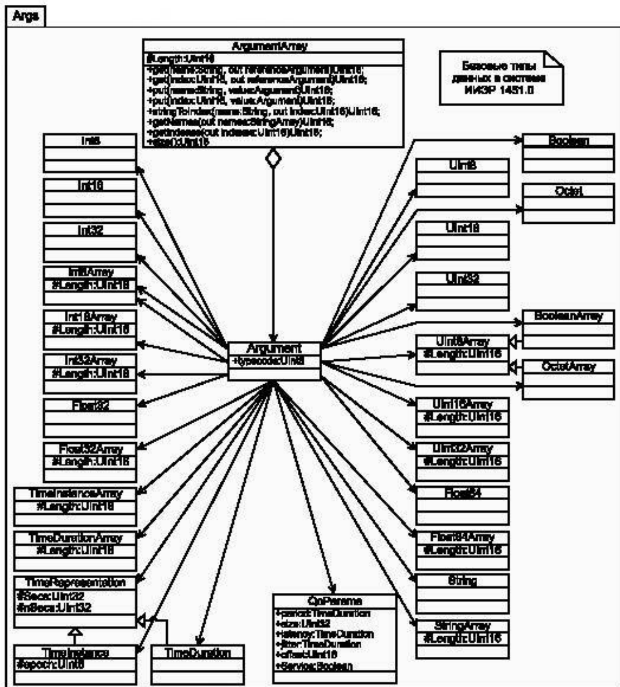
Рисунок 22 — Аргументы
