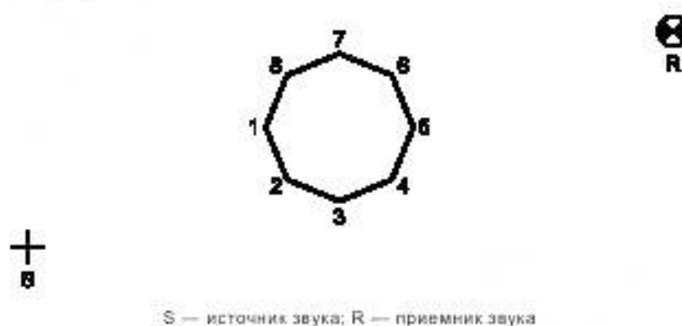
Рисунок 16 — Экранирующее здание призматической формы между источником и приемником, расположенным на малой высоте
