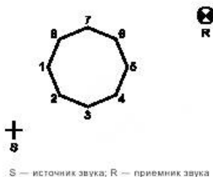
Рисунок 20 — Плоская поверхность с однородными акустическими свойствами и здание призматической формы, приемник на большой высоте
