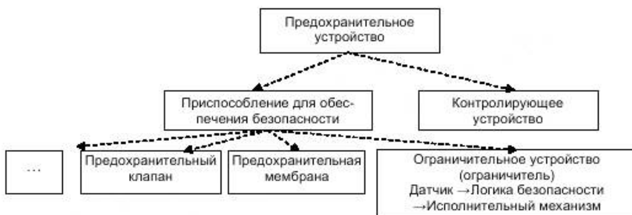
Рисунок 1 – Предохранительные устройства и устройства безопасности в соответствии с Техническим регламентом Таможенного союза «О безопасности оборудования, работающего под избыточным давлением»
