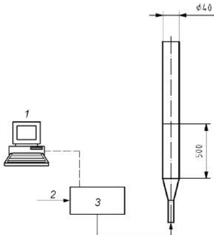
1 – регистратор данных; 2 – воздушный поток; 3 – поток материала
