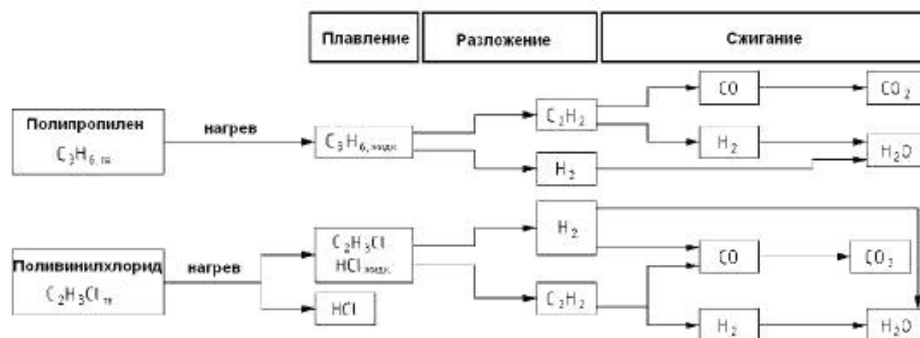
Рисунок 4 — Модель горения пластмасс
