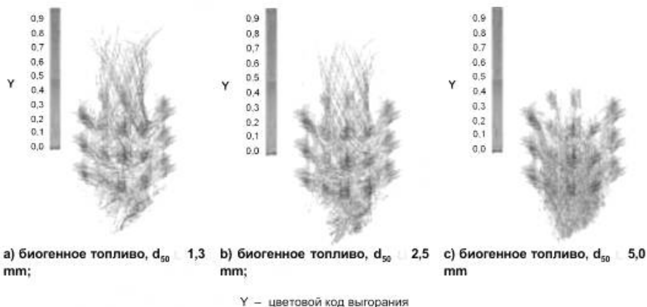
Рисунок 6 — Симуляция выгорания ТВТ в котле
