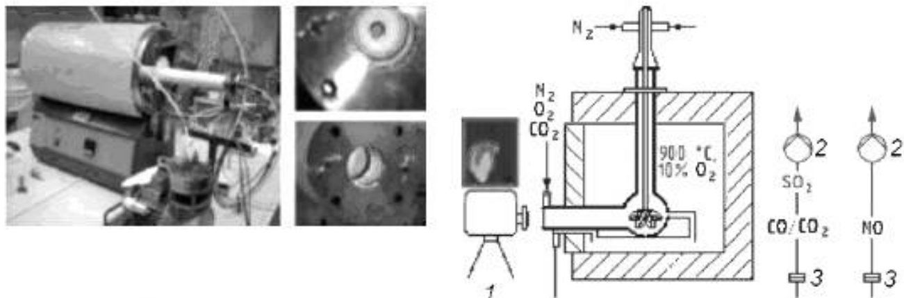
1 – камера высокого разрешения; 2 – насос; 3 – фильтр
