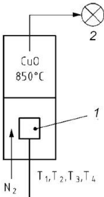
1 – проба; 2 – определение \text{CO}_2 в режиме реального времени
