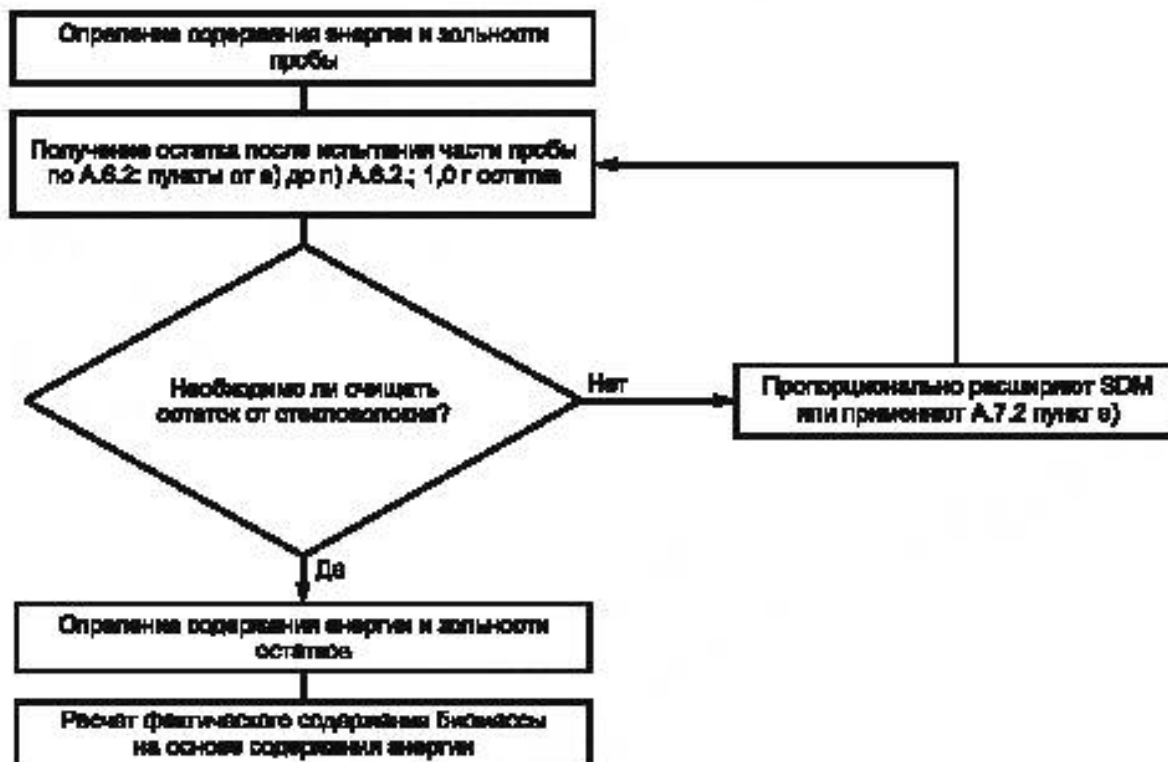
Рисунок А.2 – Определение содержания энергии фракций биомассы и не биомассы
