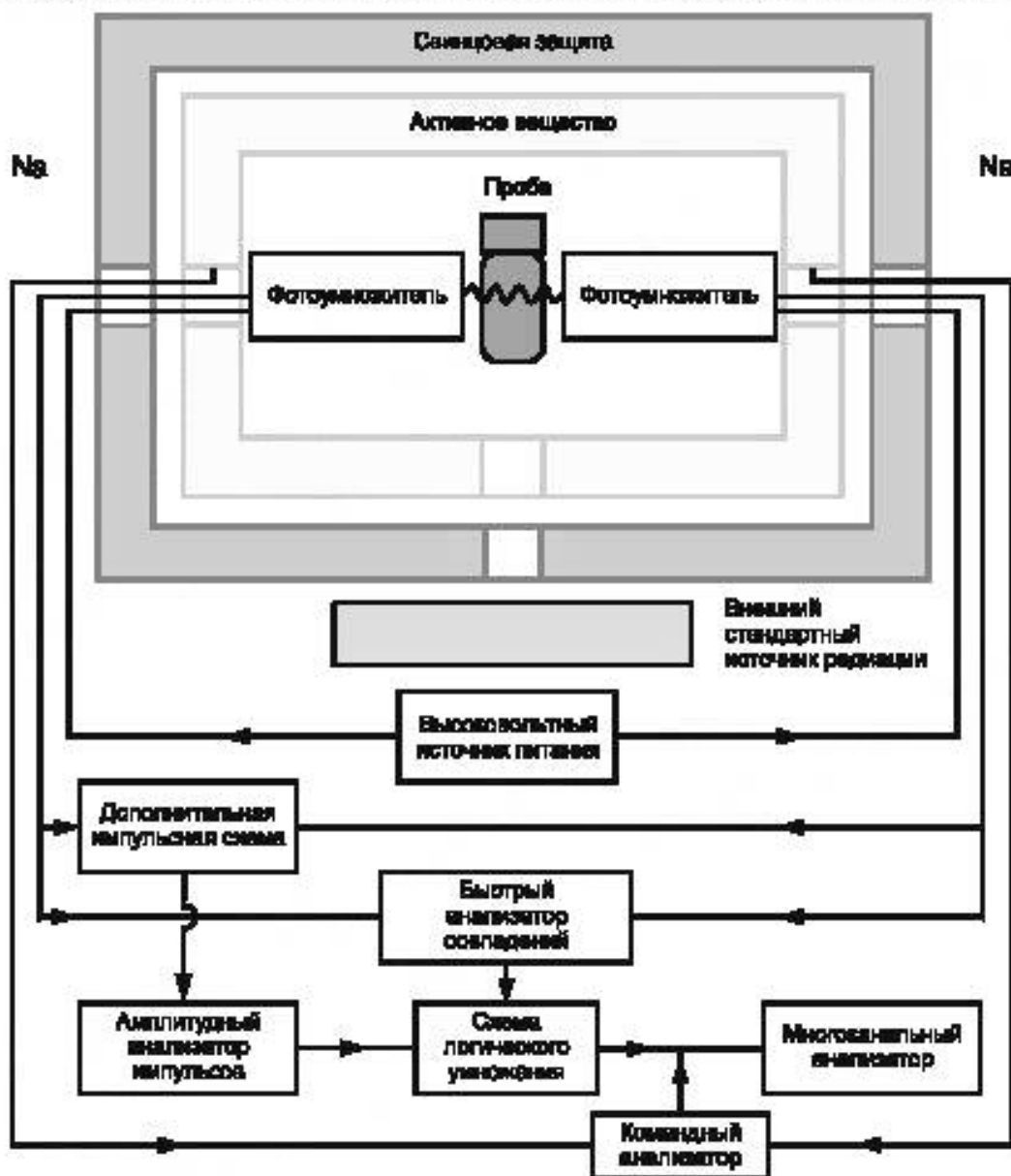
Рисунок С.1 – Жидкостной сцинтилляционный счетчик
