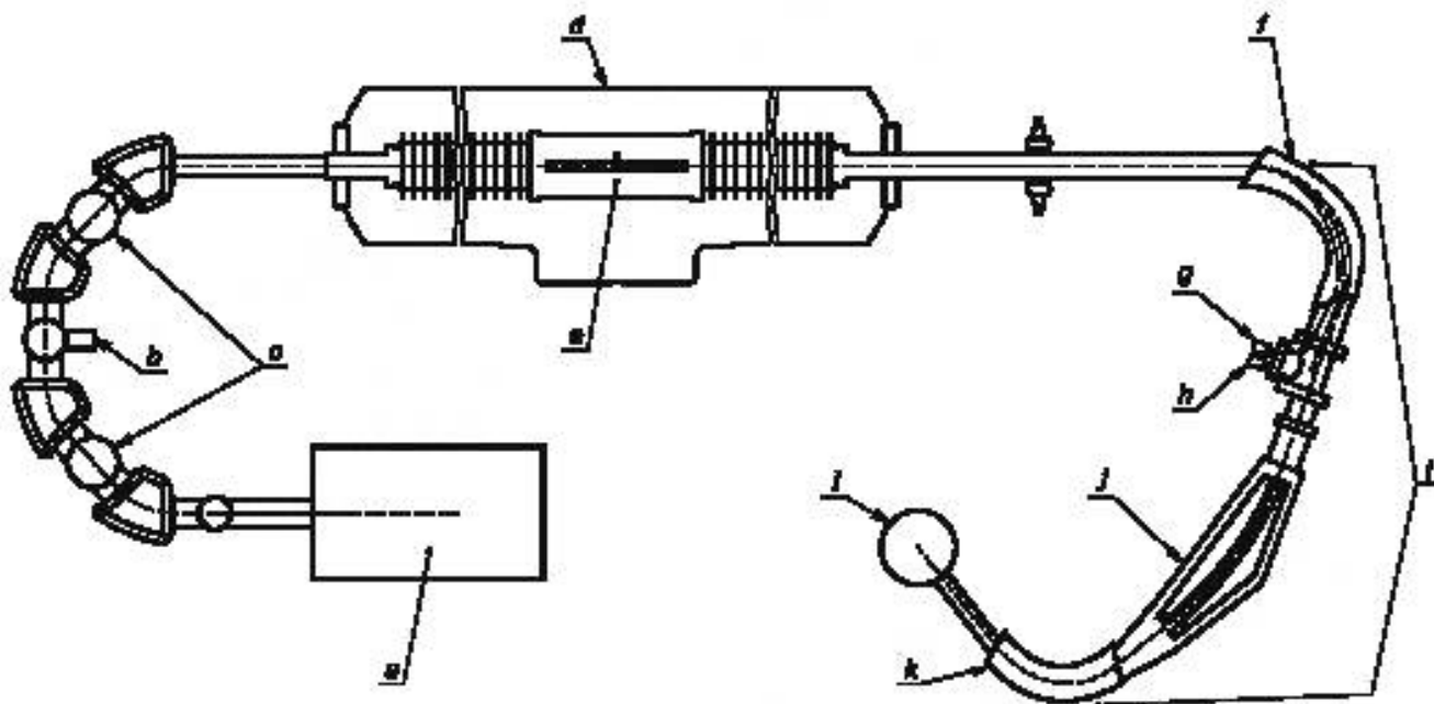
a – источник ионов на 59 проб; b – прерыватель; c – рекомбинатор; d – такедмный ускоритель; e – защищенный канал; f – магнит 110 °C; g – приемник ^{12}\text{C} ; h – приемник ^{13}\text{C} ; i – высокоэнергетический масс спектрометр; j – электростатический детектор 33 °C; k – магнит 90 °C; l – ионизационная камера
