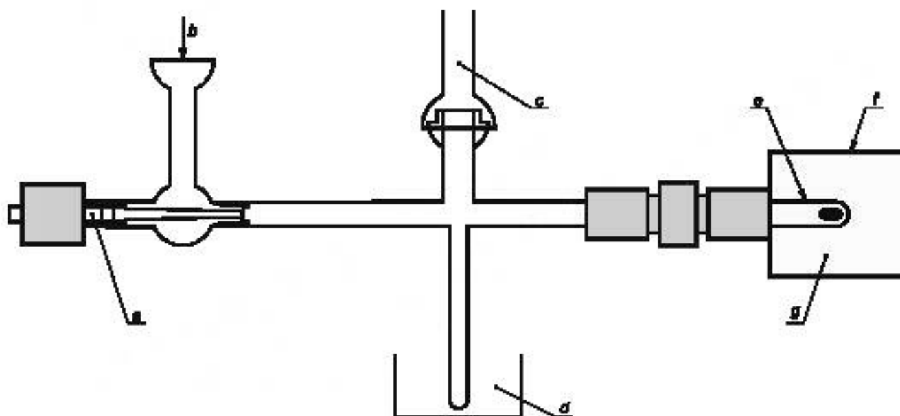
а – ампула с пробой в виде CO 2 ; б – H 2 ; с – датчик давления; д – электронный охлаждающий элемент (-18 °C для улавливания H 2 O); е – кварцевая трубка; ф – графитовая печь (800 °C); г – порошок Fe
