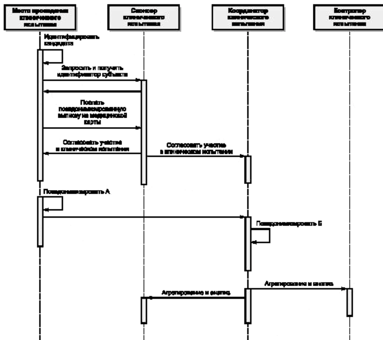
Рисунок В.9 — Псевдонимизация субъектов клинических испытаний
