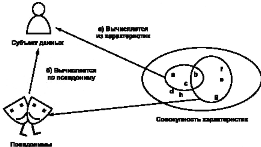
Рисунок 5 — Обратимая псевдонимизация
