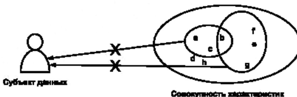
Рисунок 3 — Обезличивание
