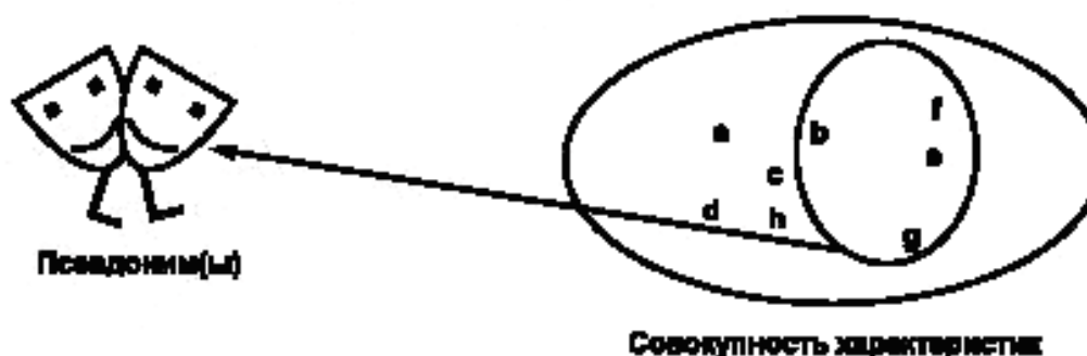
Рисунок 4 — Псевдонимизация
