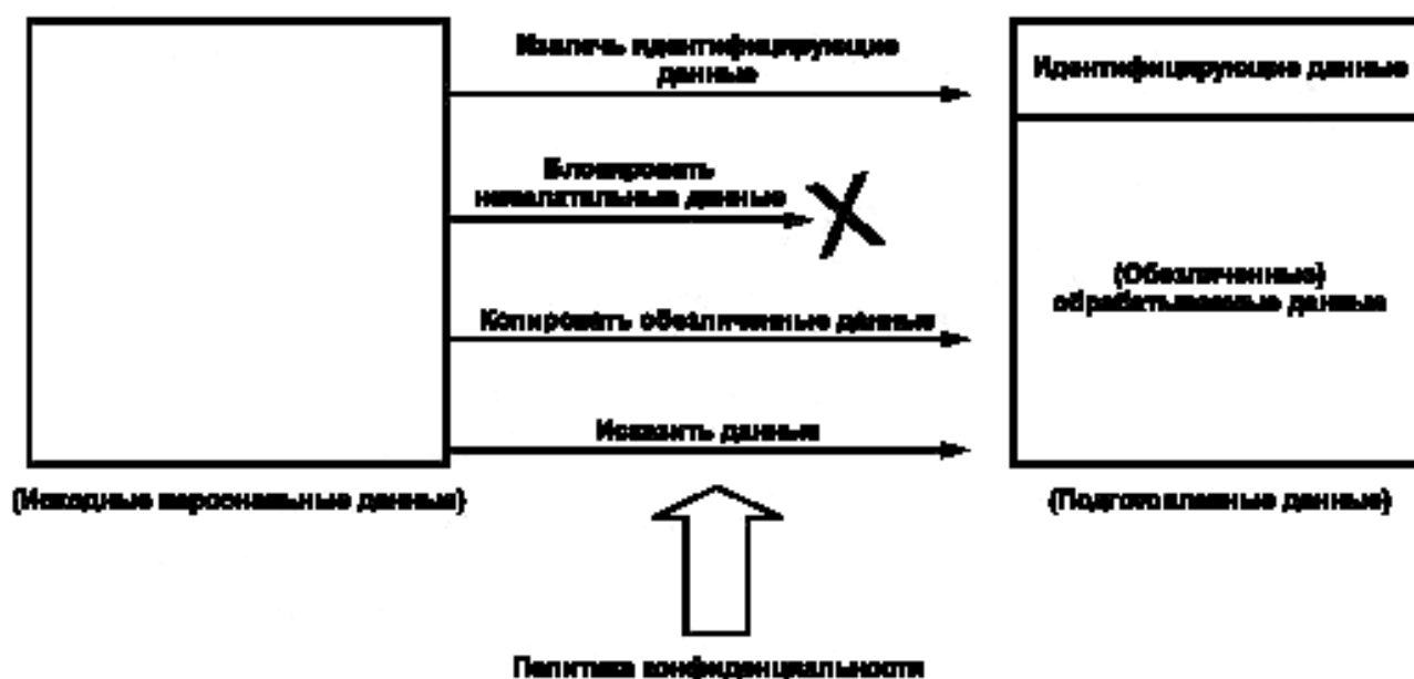
Рисунок 8 — Подготовка данных
