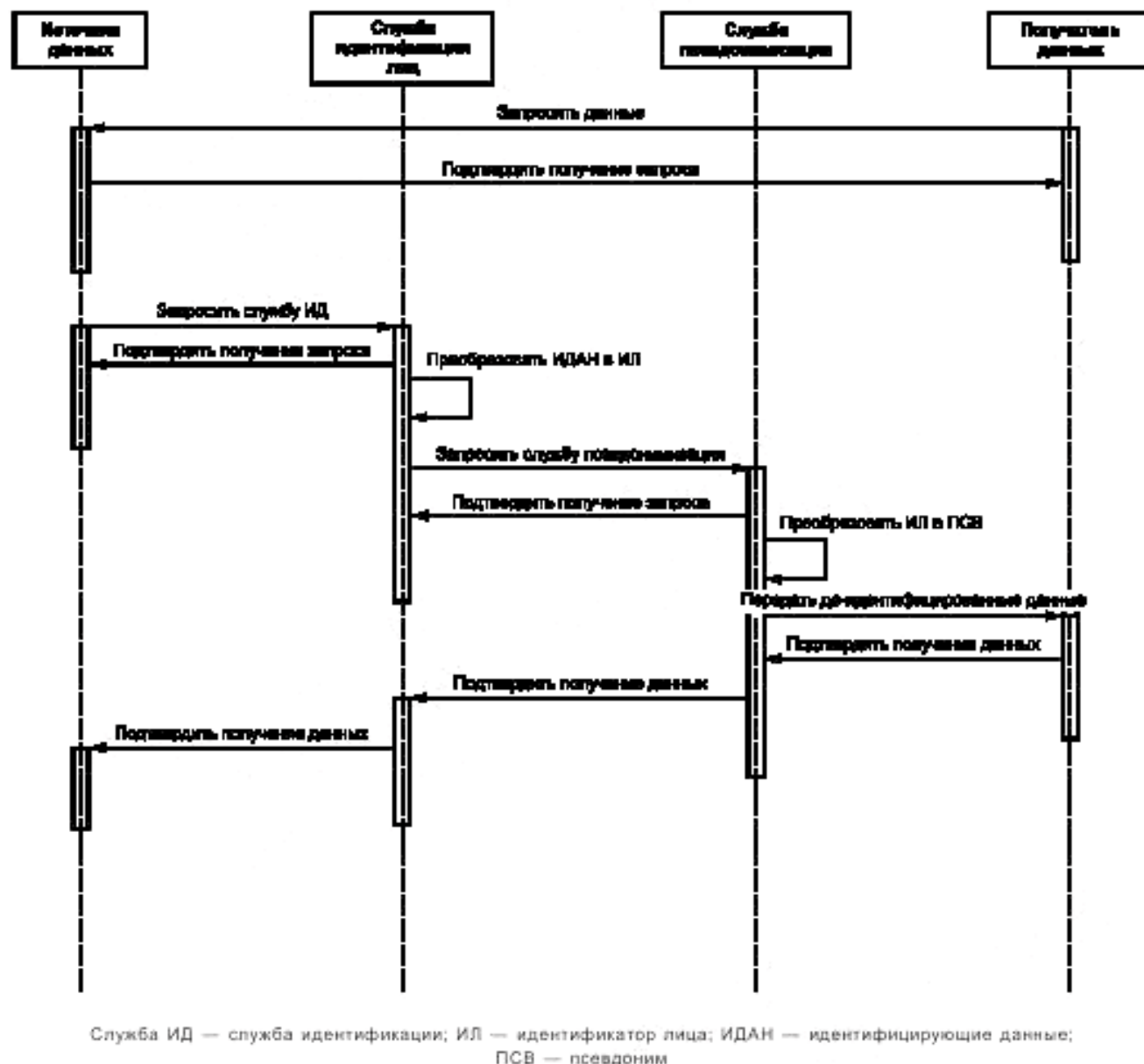
Рисунок 7 — Потоки данных
