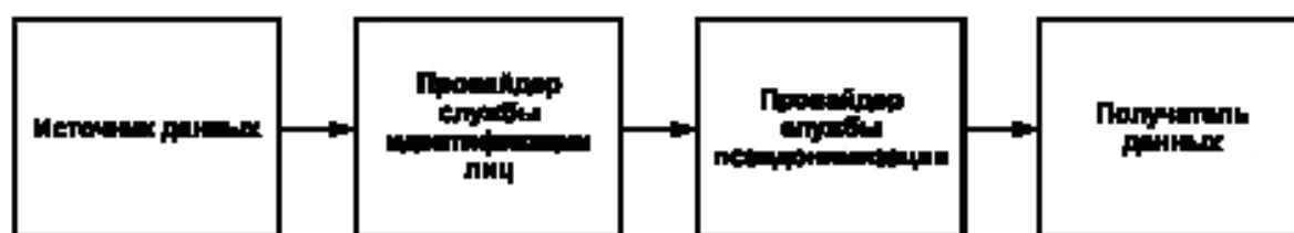
Рисунок 6 — Моделируемые сущности
