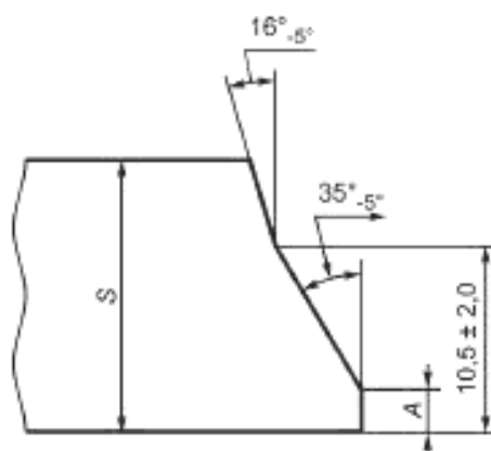
A — ширина торцевого притупления, S — толщина стенки
