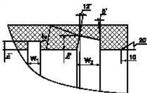
Рисунок 1 — Геометрические размеры муфты с центральным ограничителем
