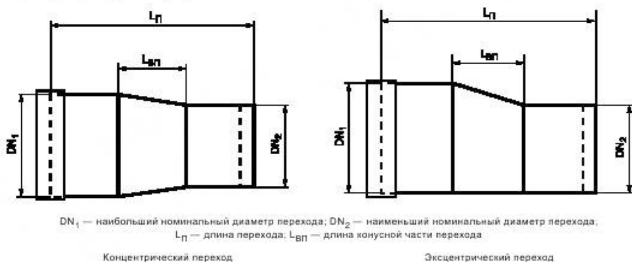
Рисунок 6 — Переходы
