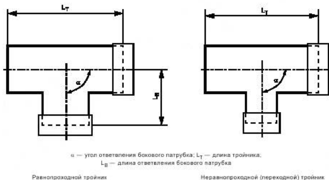
Рисунок 7 — Тройники
