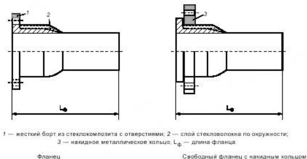
Рисунок 8 — Фланцы
