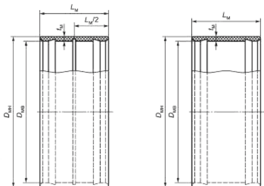
а – Муфта с центральным упором
