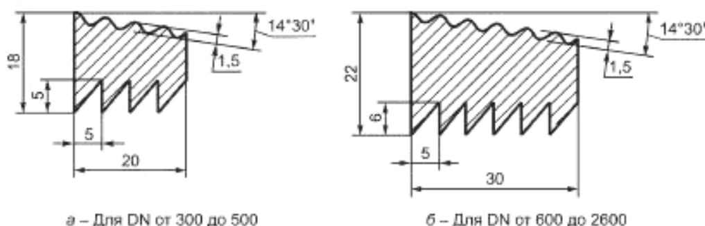
Рисунок Г.1 — Профили уплотнительных колец
