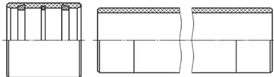
Рисунок 8 — Раздельная комплектация труб и муфт
