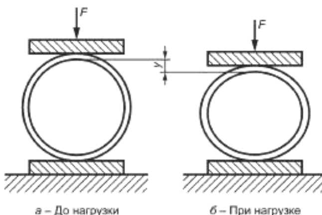
Рисунок 10 — Схема испытания на нагрузочной машине
