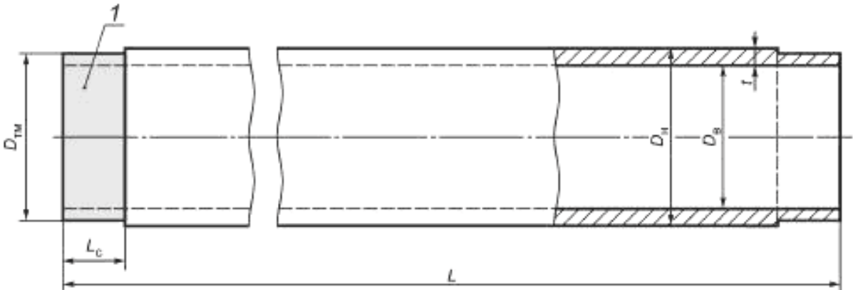
1 — калиброванная часть трубы для установки муфты; D_n — наружный диаметр; t — толщина стенки; L — длина трубы; D_{\text{тм}} — диаметр под муфтовое соединение (диаметр калиброванной части трубы); D_{\text{в}} — внутренний диаметр; L_c — длина соединения (длина калиброванной части трубы под муфтовое соединение)
