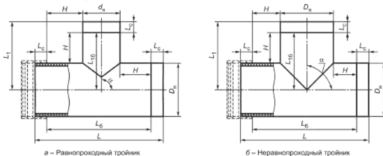
Рисунок 6 — Основные размеры тройников
