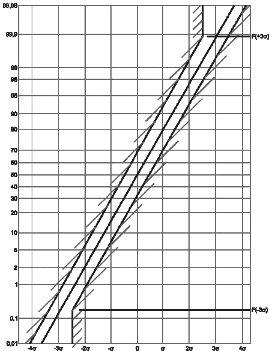
Рисунок 5 — Поля допуска для интегральной плотности распределения вероятности
