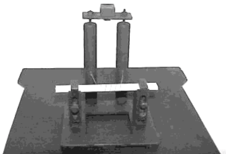
Рисунок 1 — Пример монтажа испытательного зажимного приспособления
