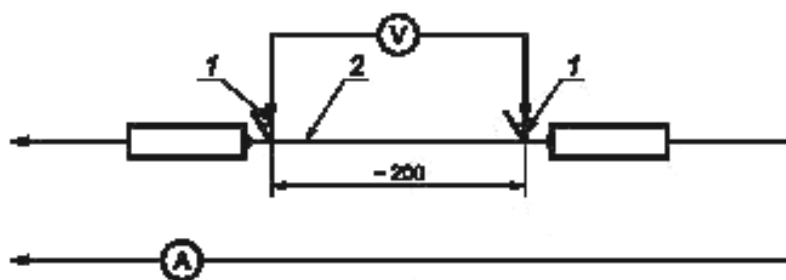
1 — зажимные измерительные щупы; 2 — испытываемая проволока
