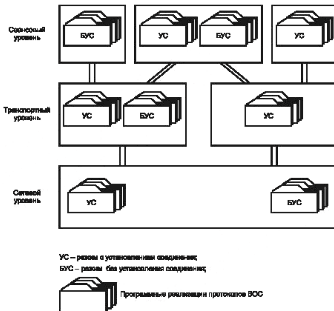
Рисунок 2b — Пример сложной реальной внутренней структуры
