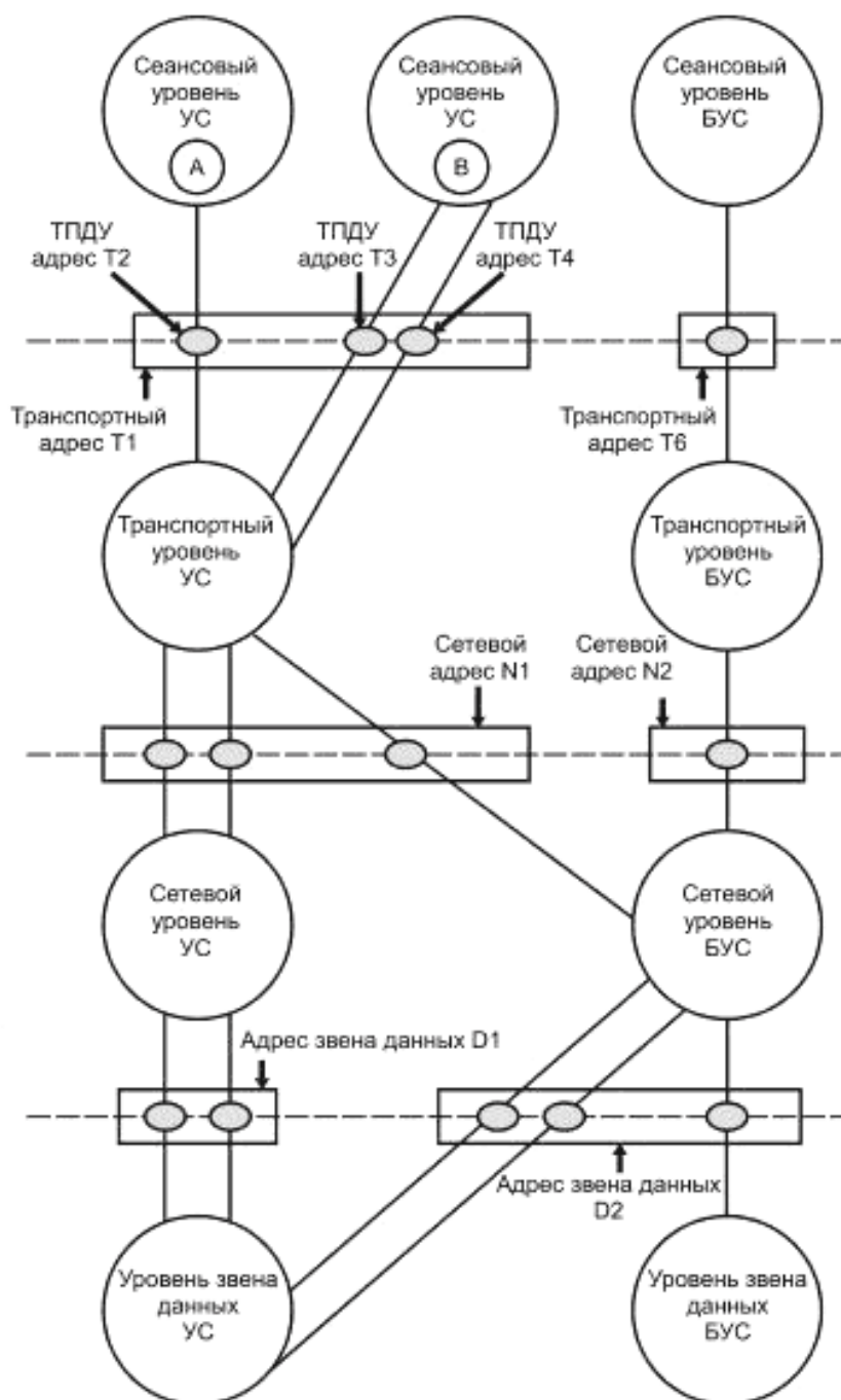
Рисунок 9 — Пример структуры адресации для уровней 2-5 системы «S»
