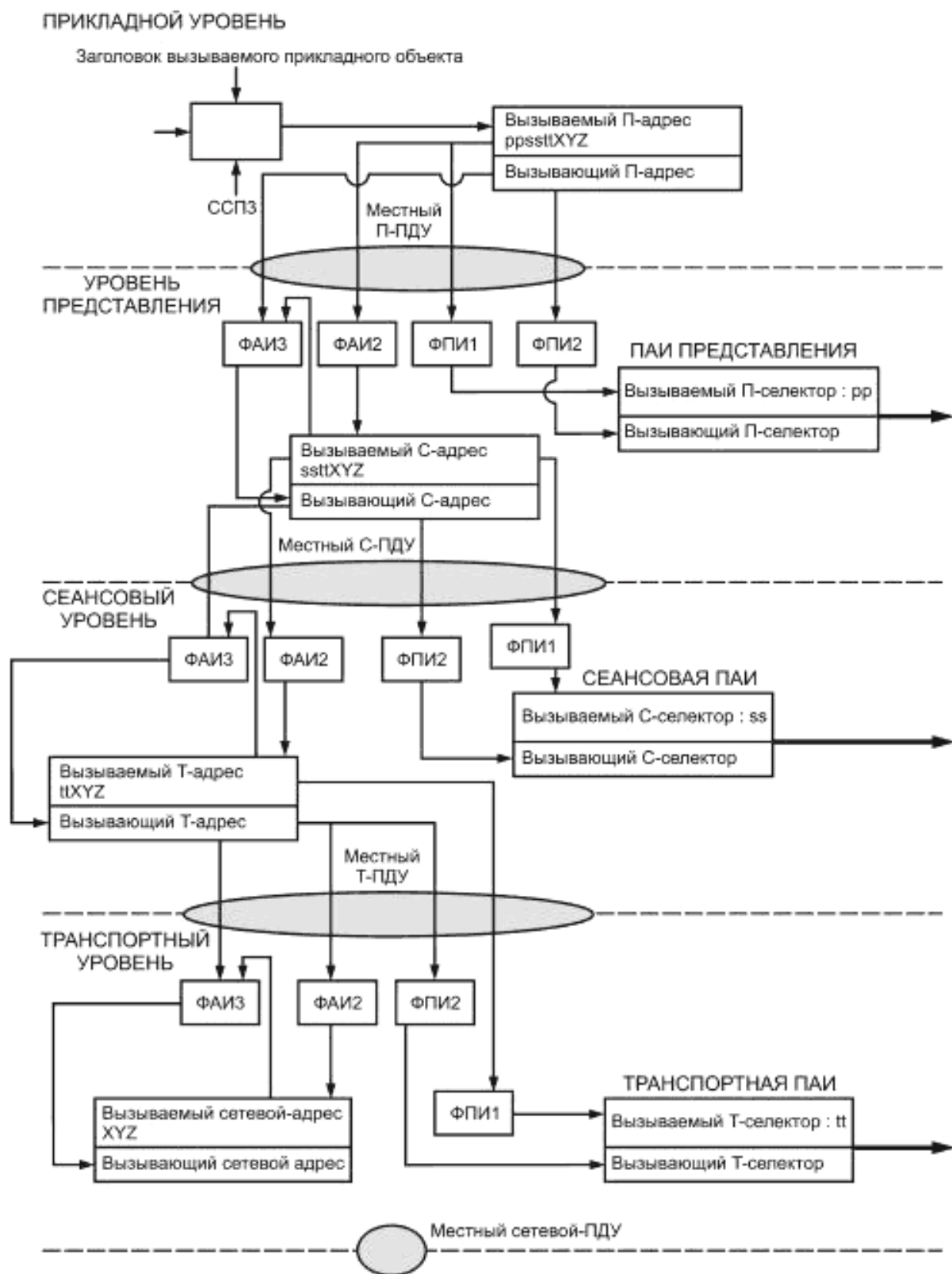
Рисунок 10 — Влияние способов инициализации в вызывающей оконечной системе
