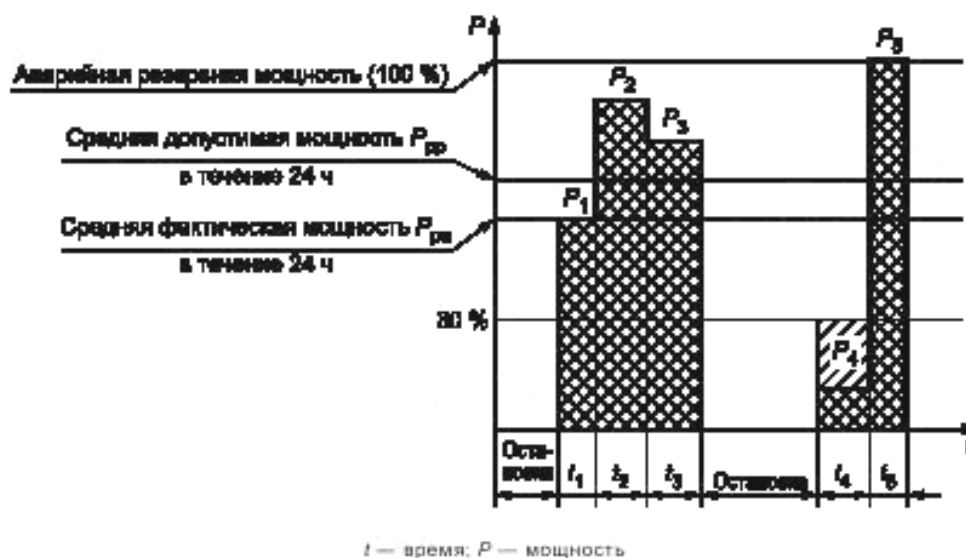
Рисунок 4 — График-иллюстрация аварийной резервной мощности (ESP)
