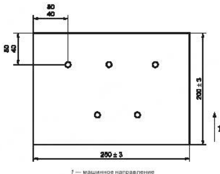
Рисунок 1 — Расположение точек на испытуемом образце для измерения средней толщины образцов
