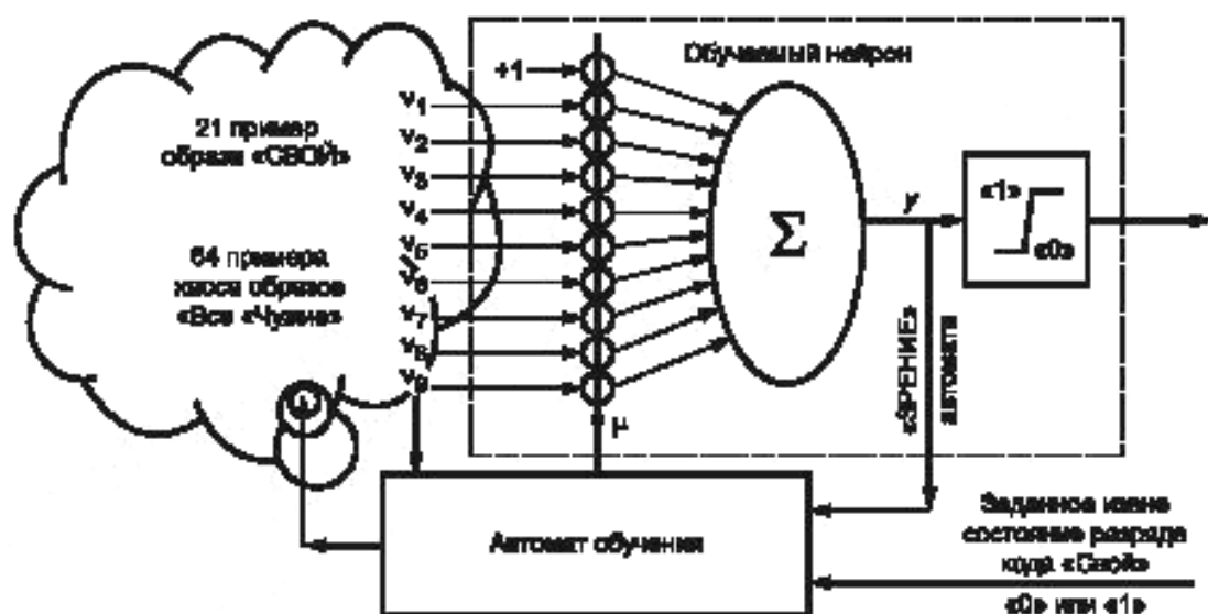
Рисунок 1 — Блок-схема обучения одного искусственного нейрона
