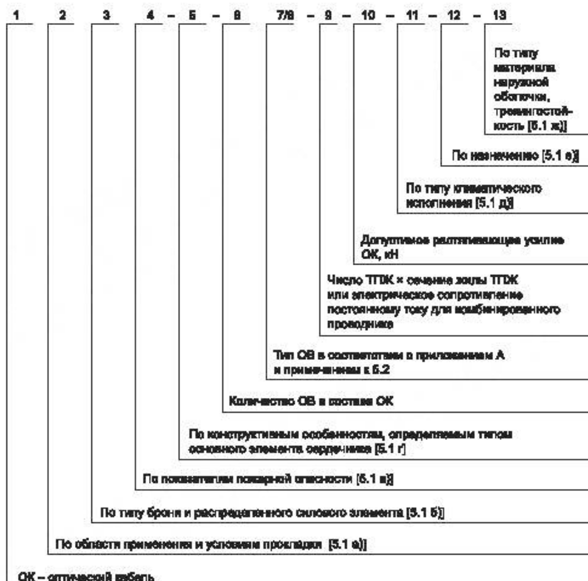
Рисунок 1 — Структура условного (кодového) обозначения оптического кабеля
