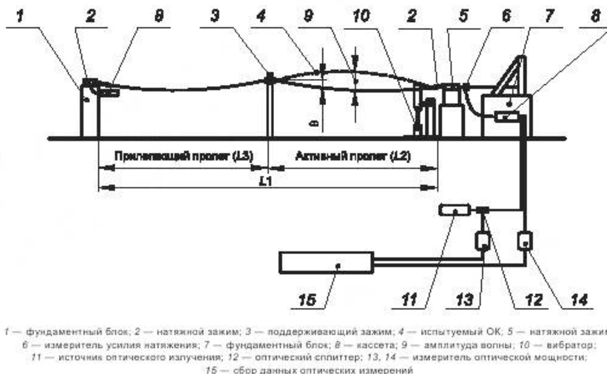
Рисунок 10 — Схема испытания ОК на воздействие галопирования
