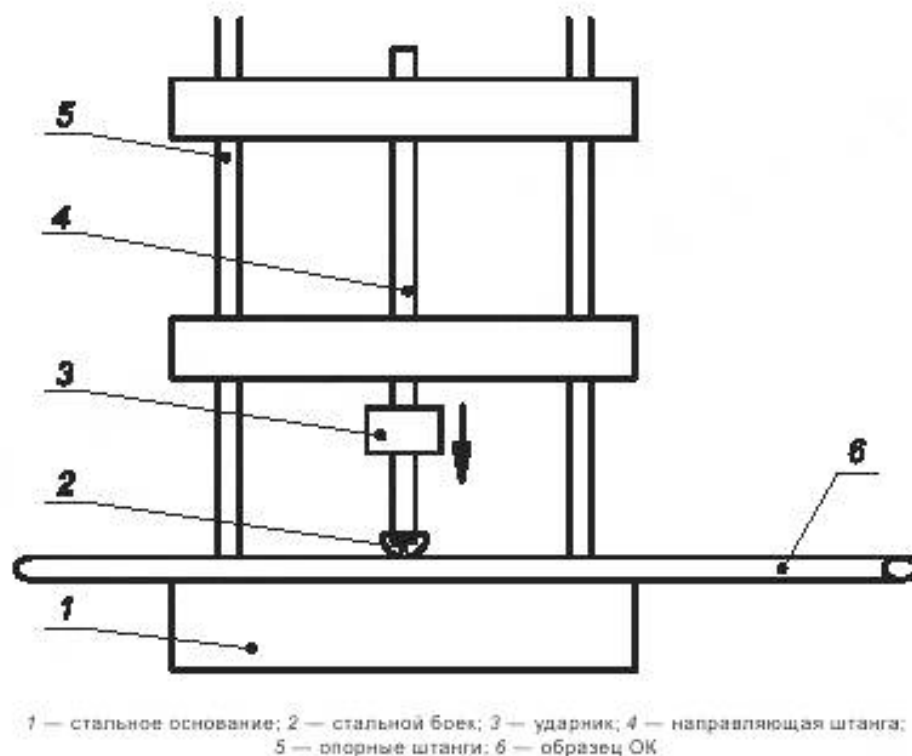
Рисунок 5 — Схема испытания ОК на воздействие удара
