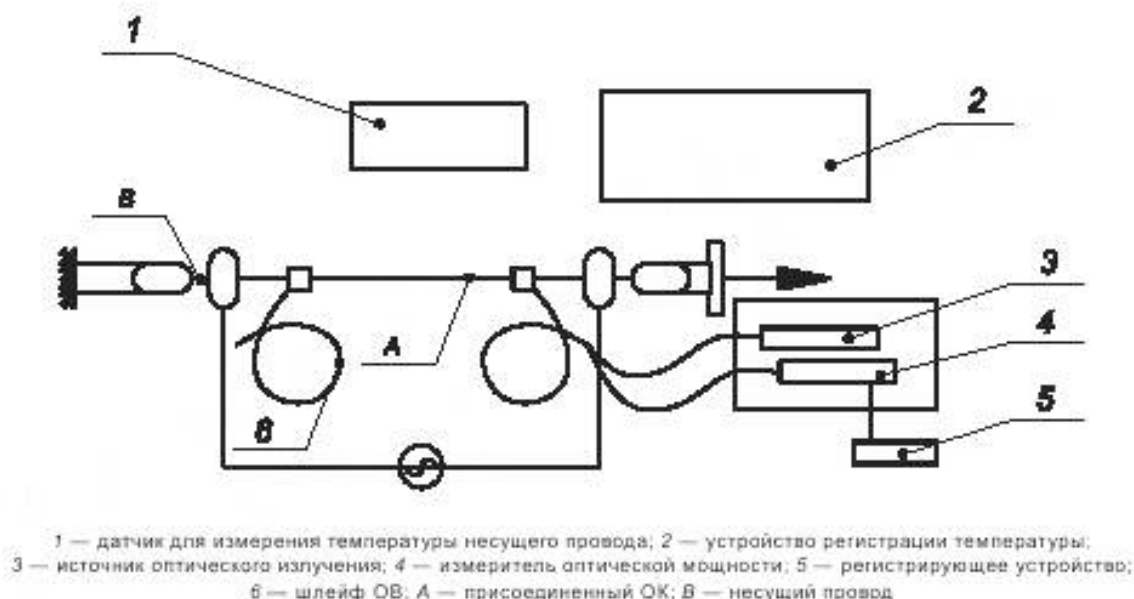
Рисунок 18 — Схема испытания ОК на протекание тока короткого замыкания ЛЭП
