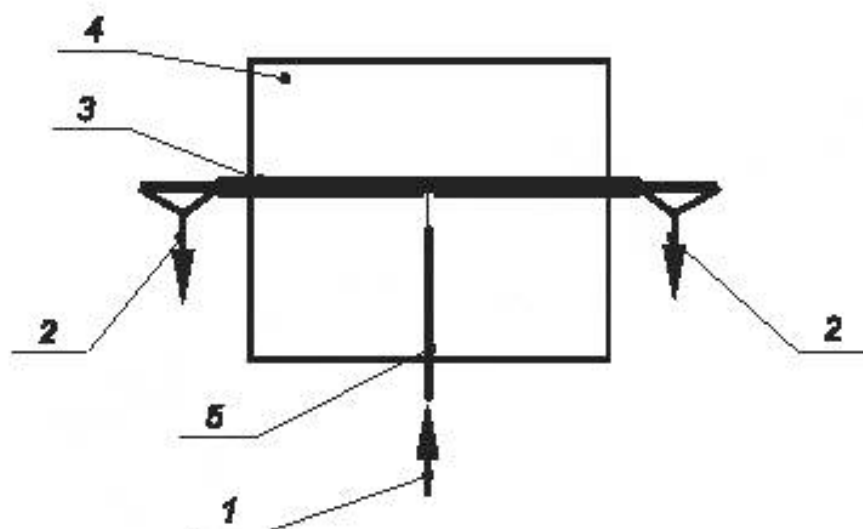
1 — ввод тока; 2 — стекание тока; 3 — образец ОК; 4 — короб с песком; 5 — металлический электрод
