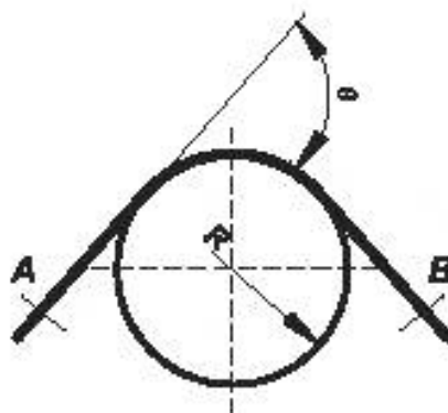
Рисунок 11 — Схема испытания ОК на перемотку через ролик
