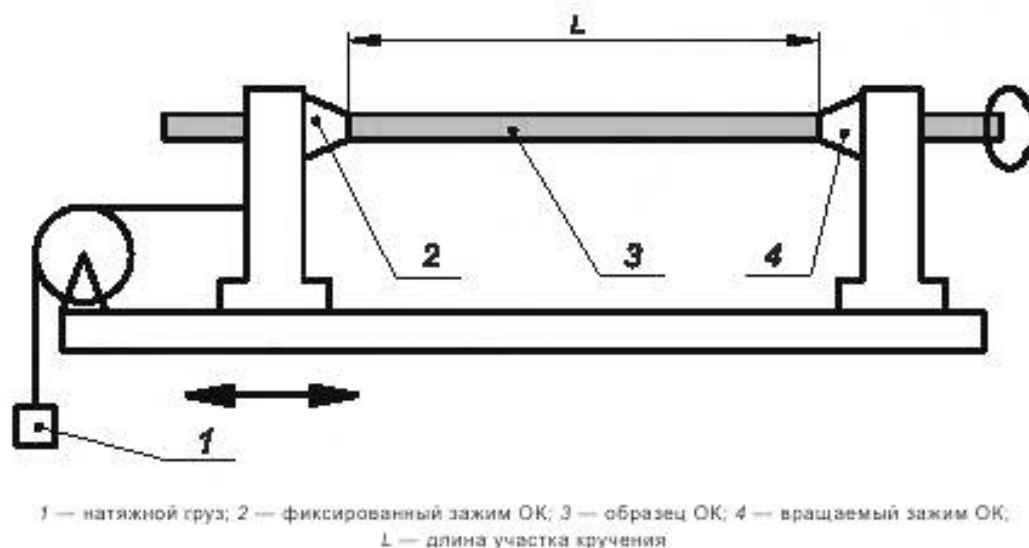
Рисунок 8 — Схема испытания ОК на воздействие осевого кручения
