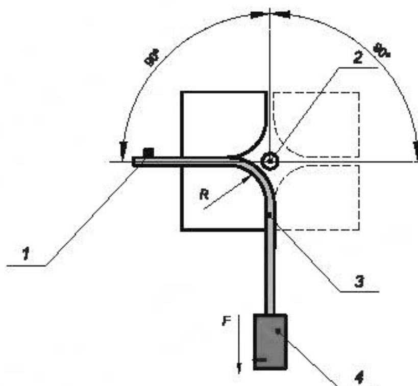
Рисунок 7 — Схема испытания ОК на воздействие многократных изгибов
