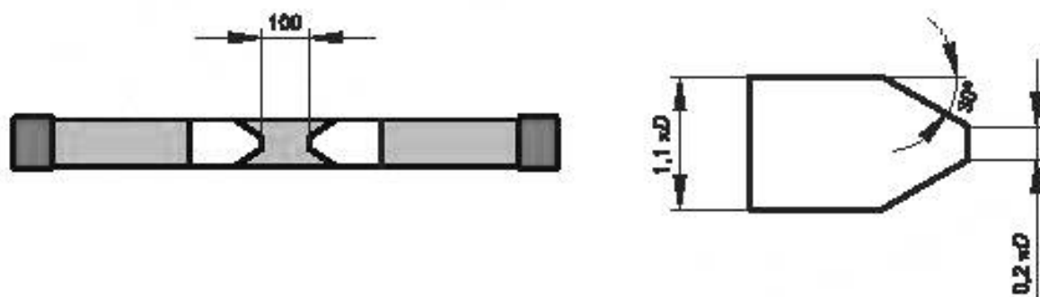
Рисунок 21 — Форма электродов, накладываемых на оболочку ОК
