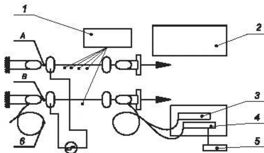
1 — датчик для измерения температуры; 2 — устройство регистрации температуры; 3 — источник оптического излучения; 4 — измеритель оптической мощности; 5 — регистрирующее устройство; 6 — шлейф ОБ; А, В — испытуемые образцы ОК
