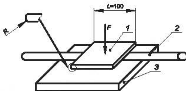
R , равный 5 мм, — радиус скругления кромок подвижной плиты; F — усилие, прикладываемое к подвижной плите в соответствии с документацией на ОК; L — длина плиты; 1 — перемещаемая плита; 2 — испытуемый образец ОК; 3 — неподвижная плита
