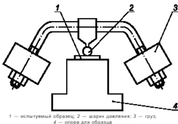
Рисунок 12а — Установка для испытания давлением шарика
