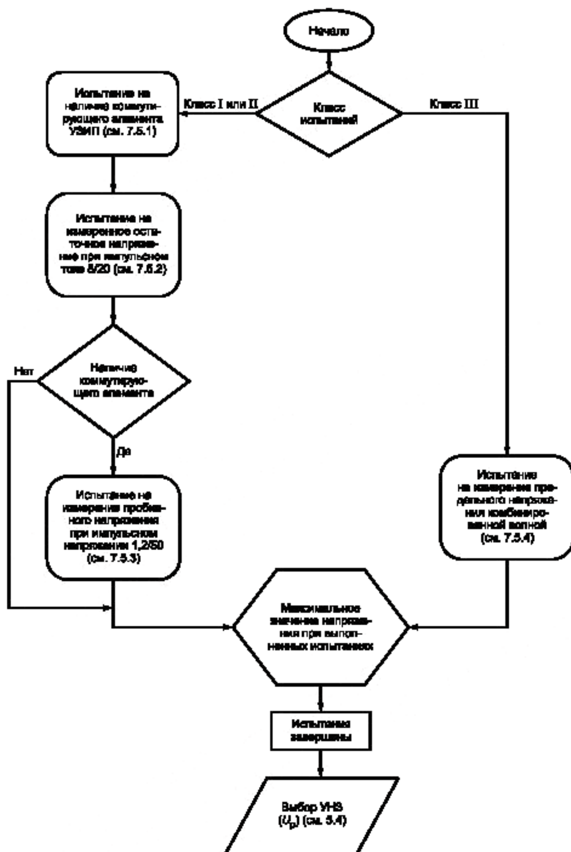
Рисунок 3 — Схема испытаний на определение уровня напряжения защиты U_{pr} (УНЗ)
