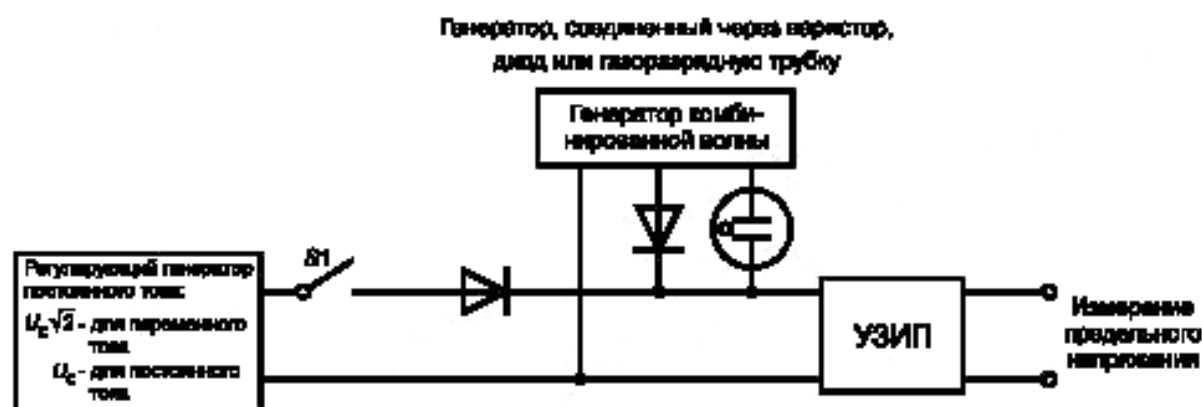
Рисунок 4 — Альтернативное испытание на измеренное предельное напряжение
