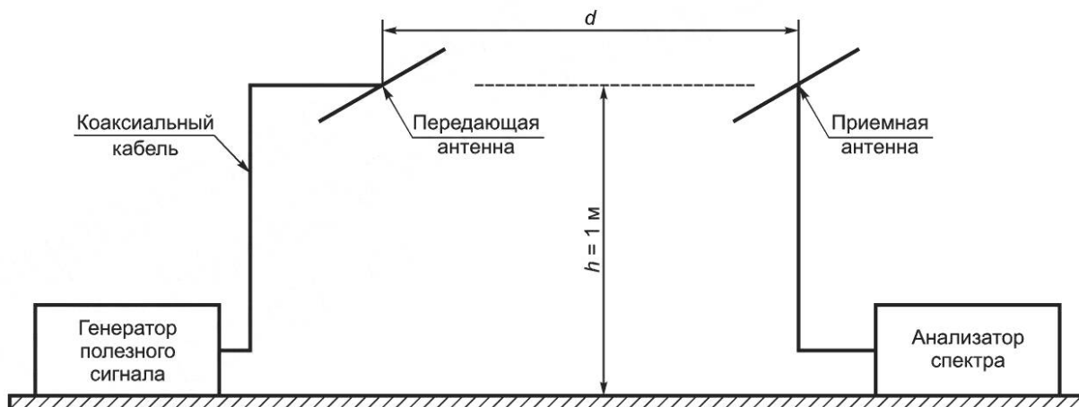
Рисунок 6 — Измерительная установка для измерений излучения методом «замещения». Второй шаг измерения
