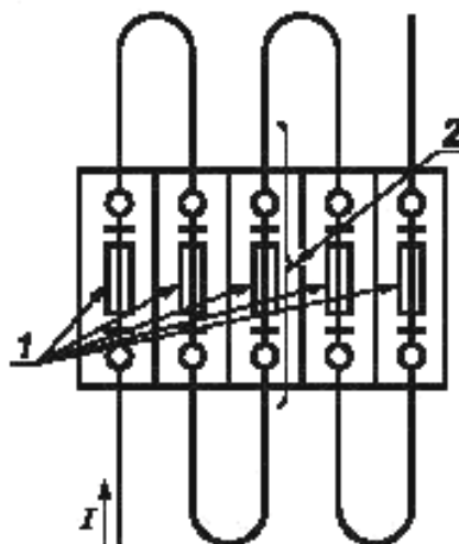
Рисунок 4 — Схема испытательного устройства при совместной установке колодок с защитой от коротких замыканий
