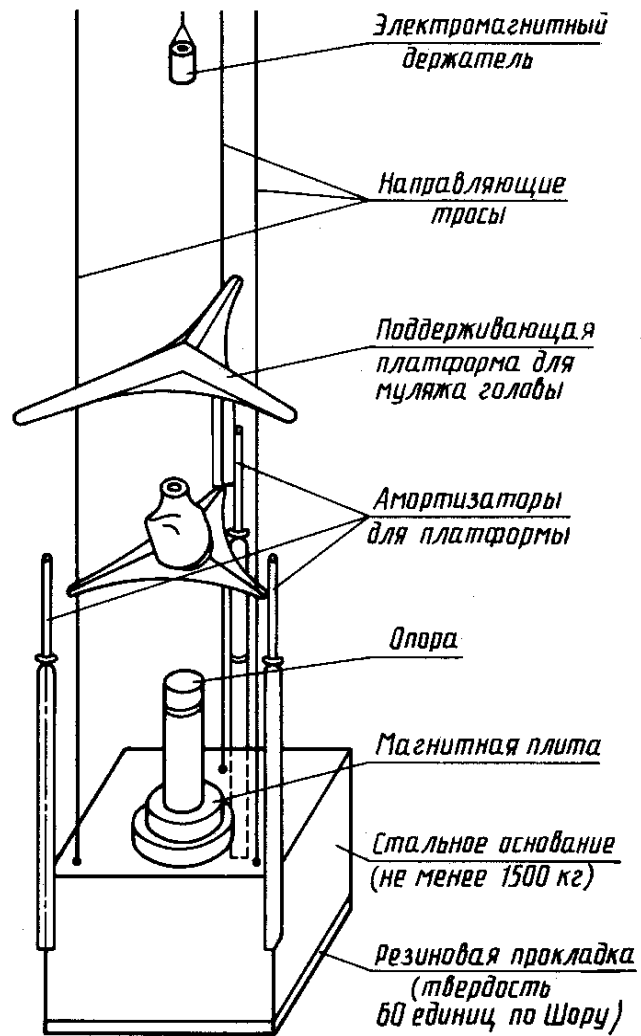
Рисунок 1а — Устройство для сброса муляжа головы
