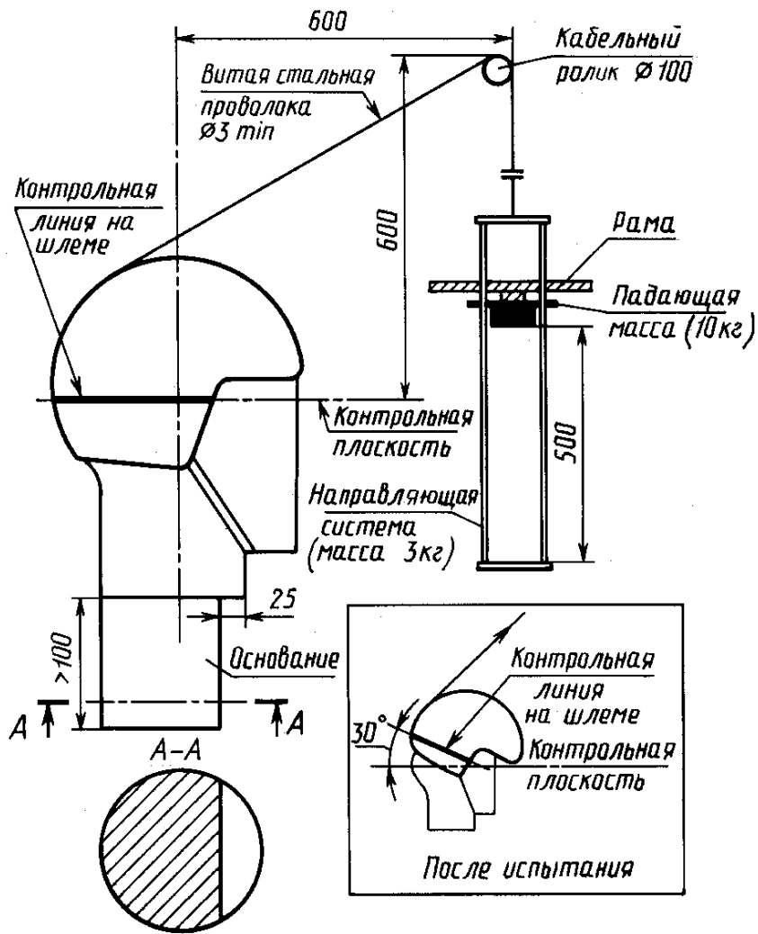
Рисунок 3 — Устройство для испытания на удержание
