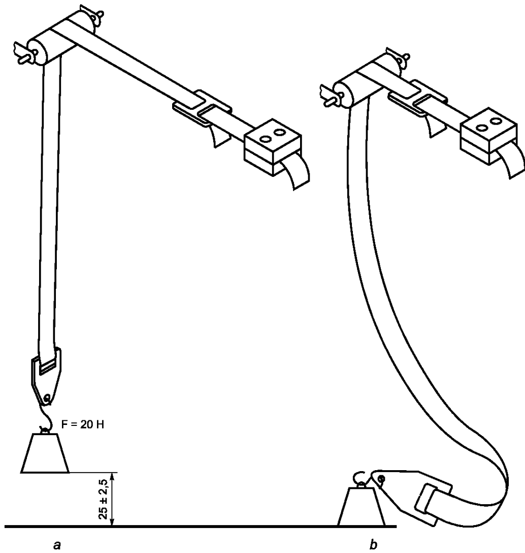
Рисунок 4 — Устройство для испытания ремешка для подбородка на проскальзывание
