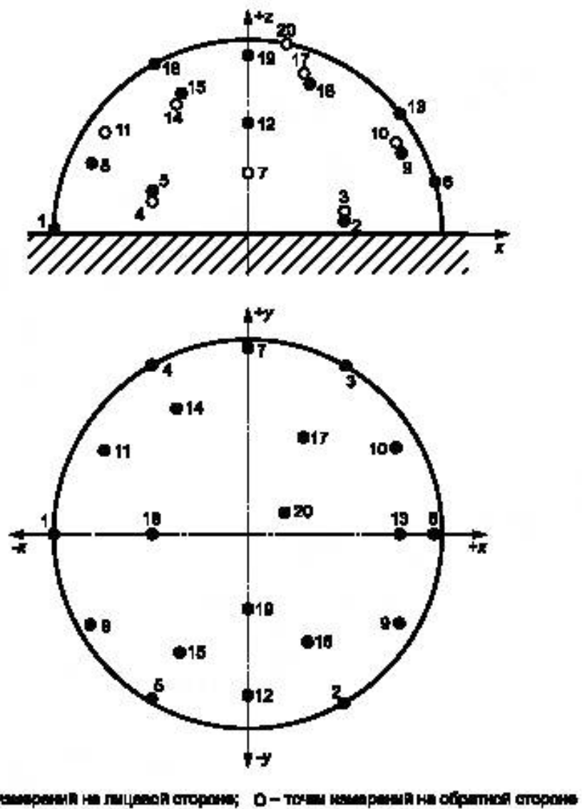
Рисунок Е.1 — Точки измерений на полусферической измерительной поверхности (общий случай)
