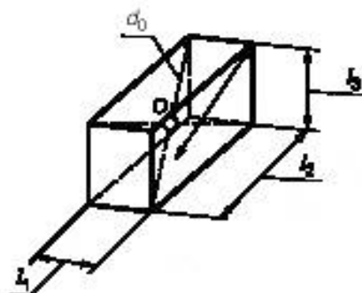
а) Заглушенная камера, d_0 = \sqrt{(l_1/2)^2 + (l_2/2)^2 + (l_3/2)^2}
