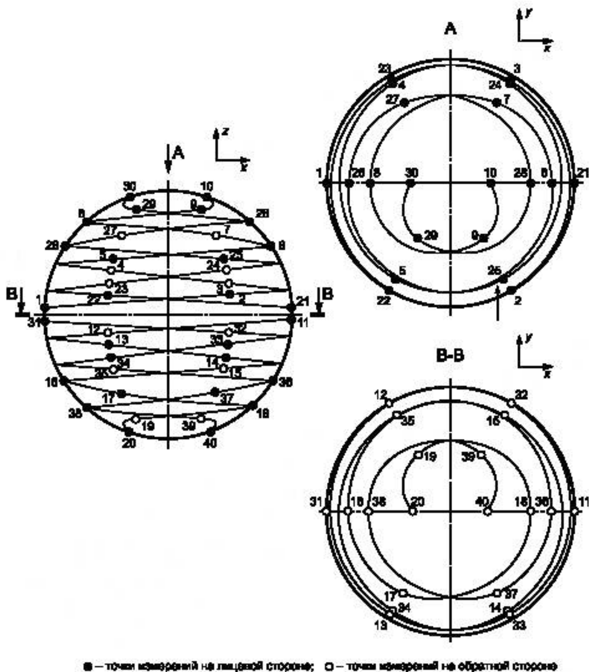
Рисунок D.1 — Точки измерений на сферической измерительной поверхности
