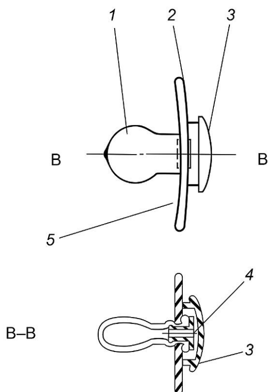
Рисунок 10 — Соска-пустышка с комбинированной пробкой, крышкой и головкой
