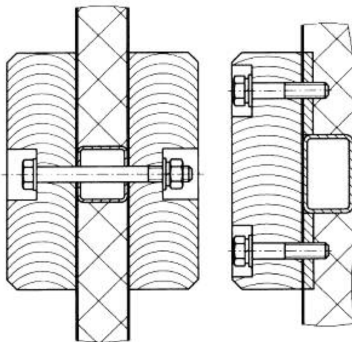
Рисунок 3 — Примеры крепления спинок сидений спецконтингента
