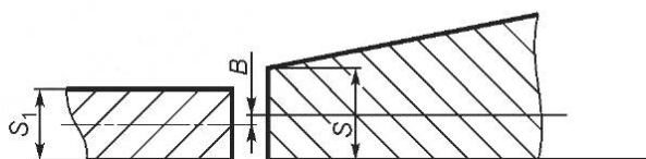
Рисунок 12.2 – Смещение кромок листов в стыковых продольных соединениях
