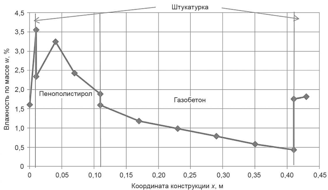
Рисунок А.1 — Распределение влажности внутри конструкции
