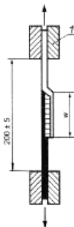
1 – зажим; w – ширина клеевого соединения
