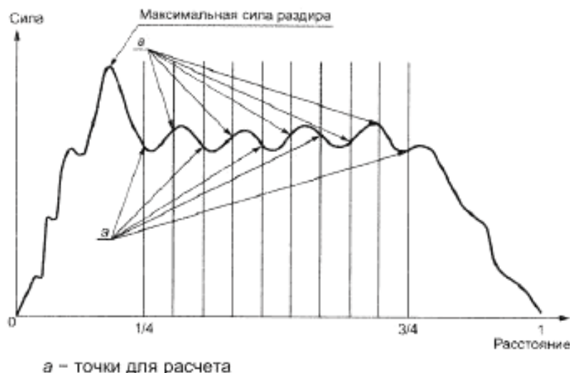
Рисунок 3 – Пример графического расчета сопротивления раздиру клеевого соединения
