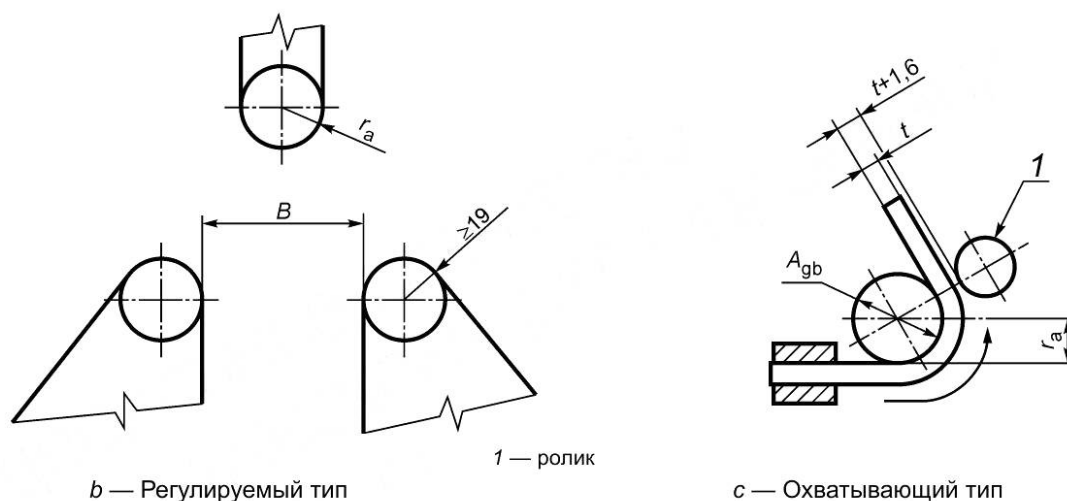
Рисунок 9, лист 2
