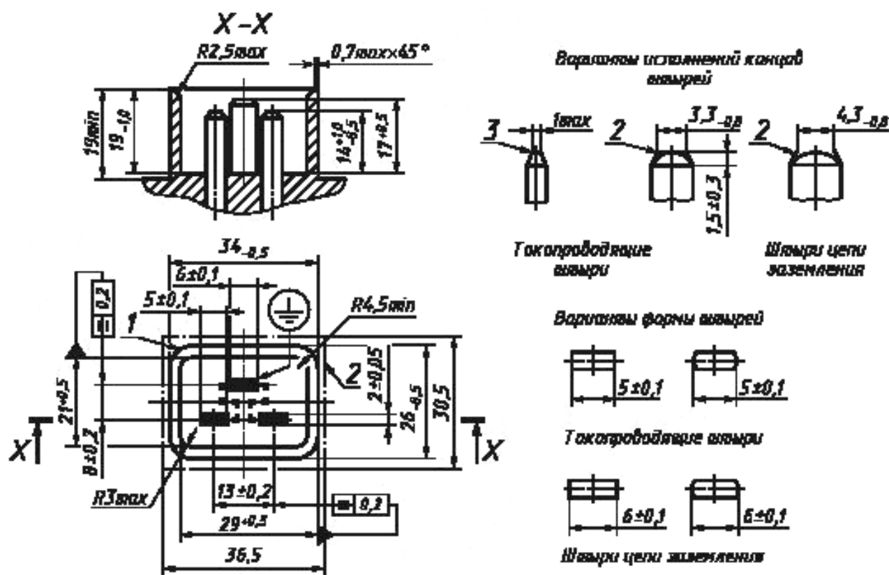
Вилка на 16 А для приборов класса I
