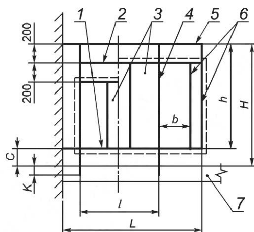
Рисунок А.3 — Решетчатые ограждения лестничных площадок
