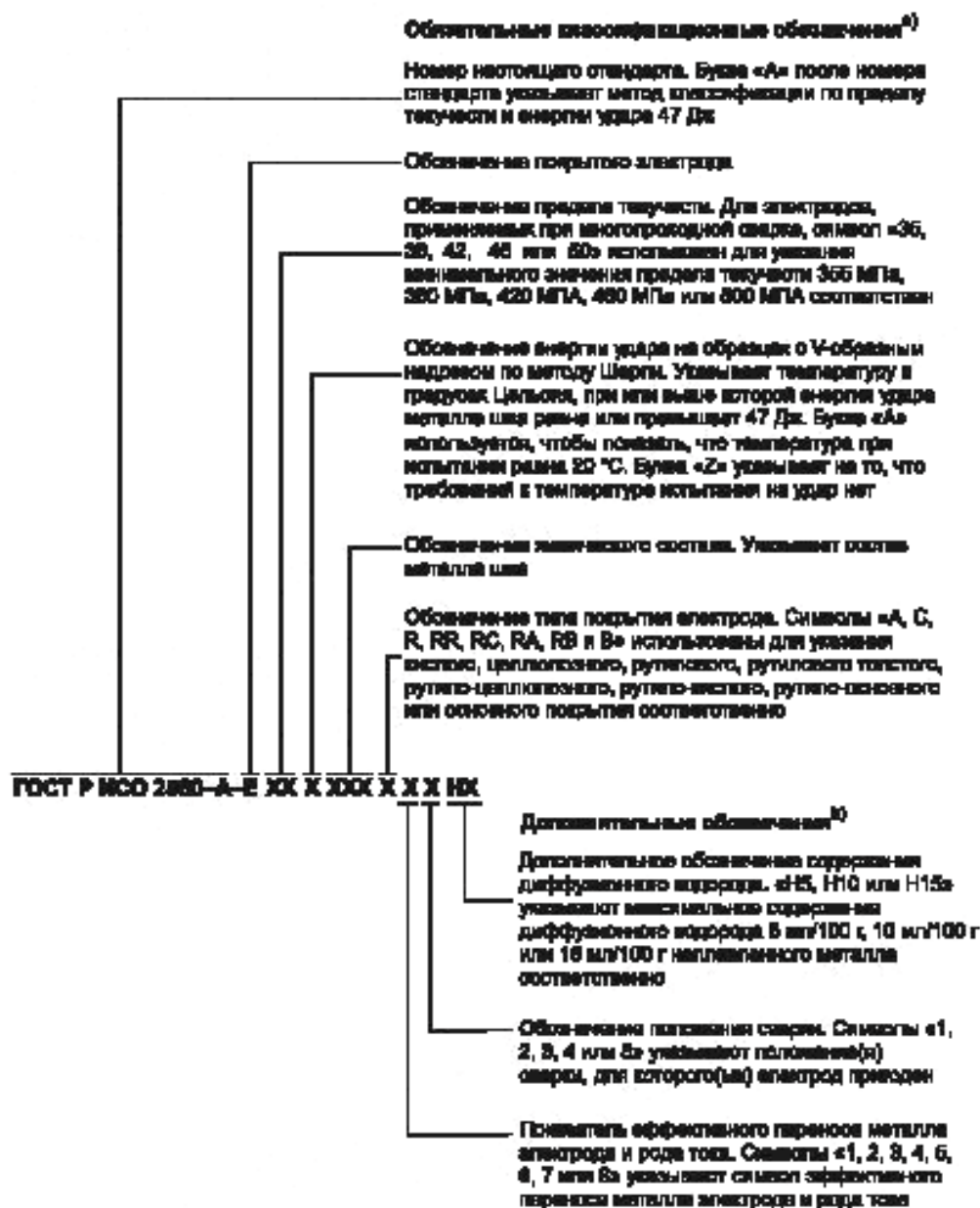
Рисунок А.1 — Обозначение электродов по ГОСТ Р ИСО 2560-A (классификация по пределу текучести и энергии удара 47 Дж)
