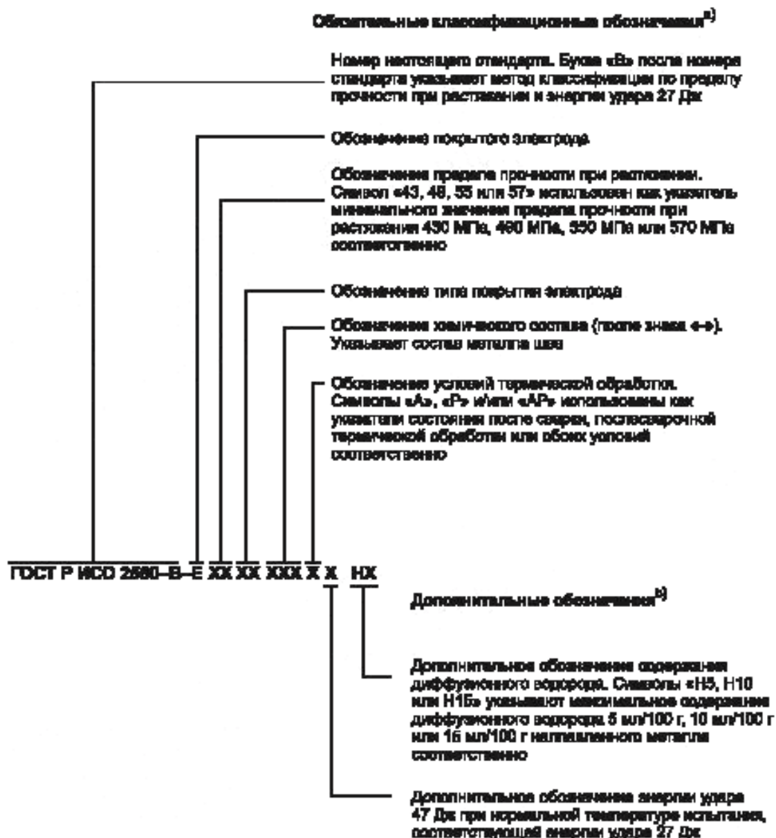
Рисунок А.2 — Обозначение электродов по ГОСТ Р ИСО 2560-B (классификация по пределу прочности при растяжении и энергии удара 27 Дж)
