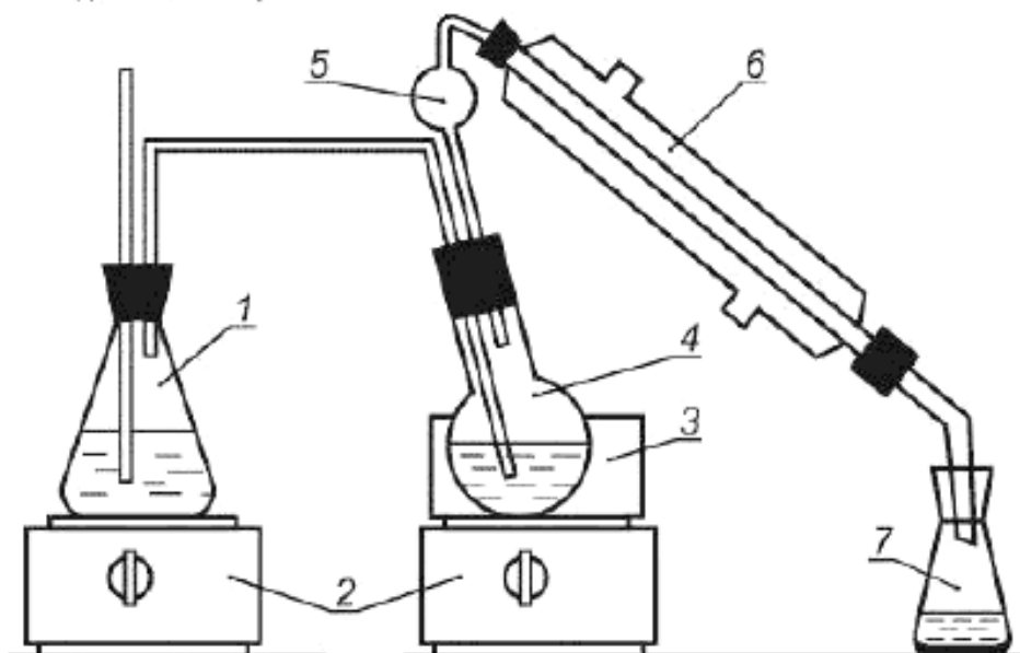
1 – паровыделитель, 2 – колбонагреватели, 3 – масляная баня, 4 – перегонная колба с продуктом, 5 – каплеуловитель, 6 – холодильник, 7 – приемная колба
