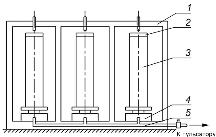
1 — рама машины; 2 — верхняя винтовая опора с оголовником; 3 — образец; 4 — гидродомкрат; 5 — маслопровод
