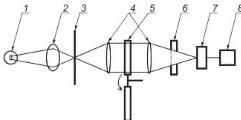
1 — источник света; 2 — объектив; 3 — щелевой ограничитель; 4 — конденсоры; 5 — светофильтры; 6 — затвор; 7 — радиометр; 8 — система, регистрирующая фототоки
