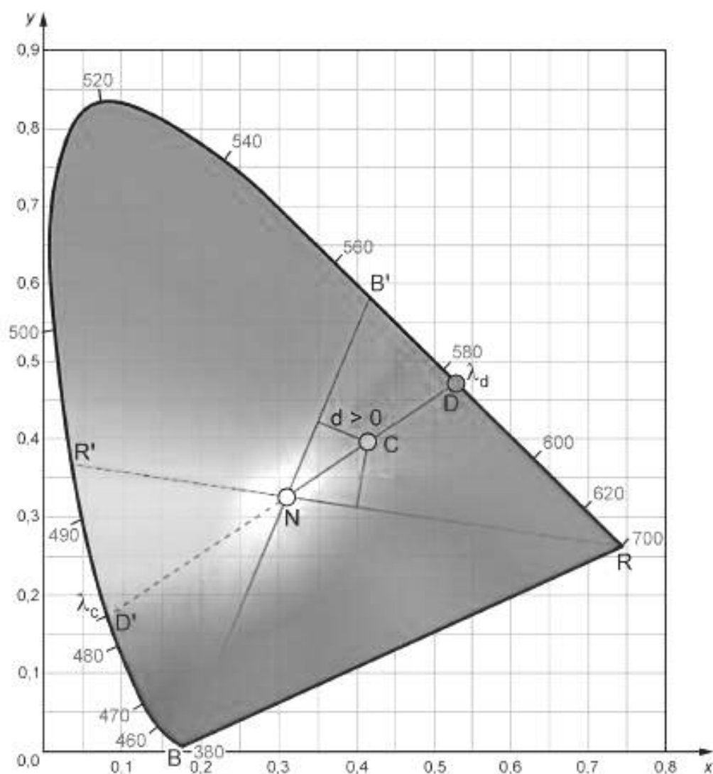
Рисунок 7 — Диаграмма цветности МКО 1931 г. и 1964 г.
