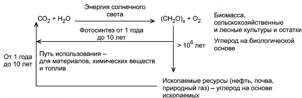
Рисунок 1 — Представление циклически полезного круговорота углерода при использовании биовозобновляемого углерода вместо углеродного сырья на основе ископаемых
