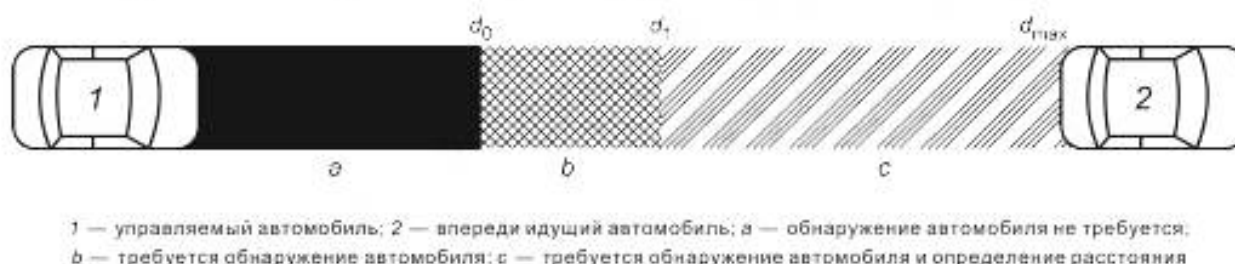
Рисунок 4 — Дальность обнаружения
