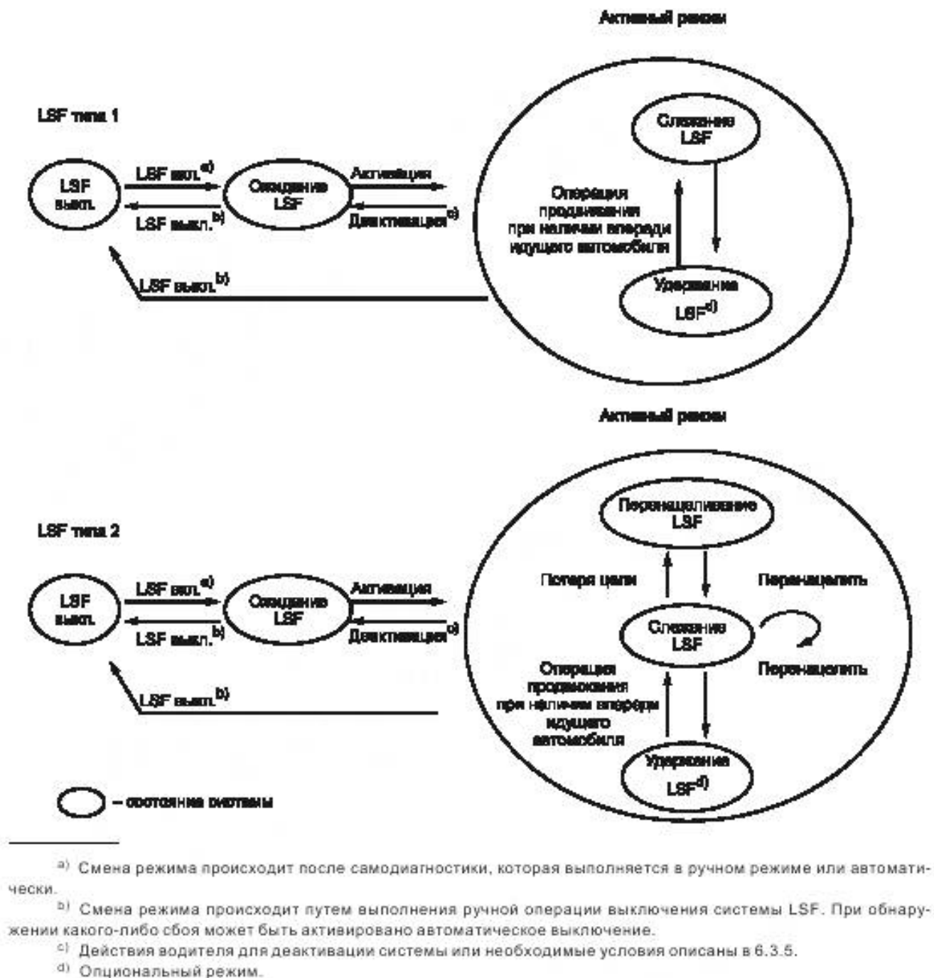
Рисунок 3 — Режимы системы LSF и их смена
