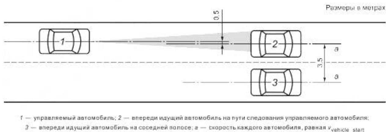
Рисунок 11 — Тестирование на выбор цели (начальные условия)
