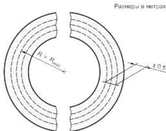
Рисунок 18 — Схема испытательного участка
