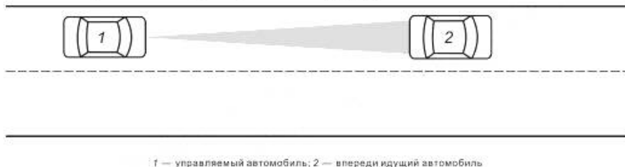
Рисунок 13 — Тестирование автоматического торможения (начальные условия)
