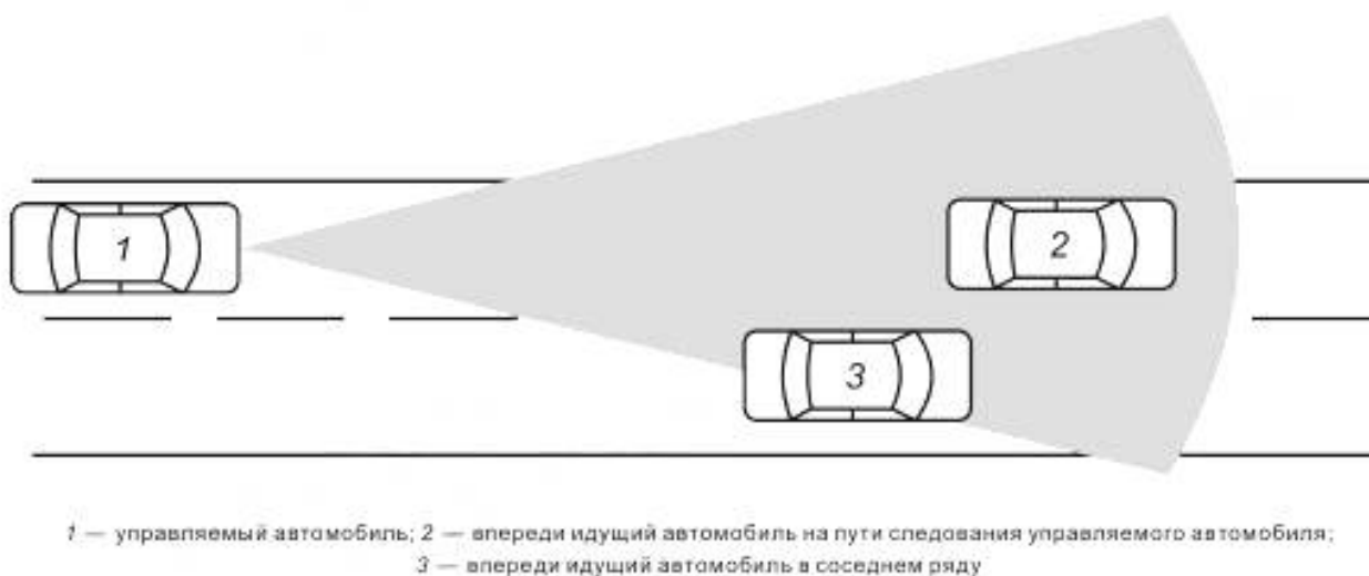
Рисунок 5 — Выбор цели
