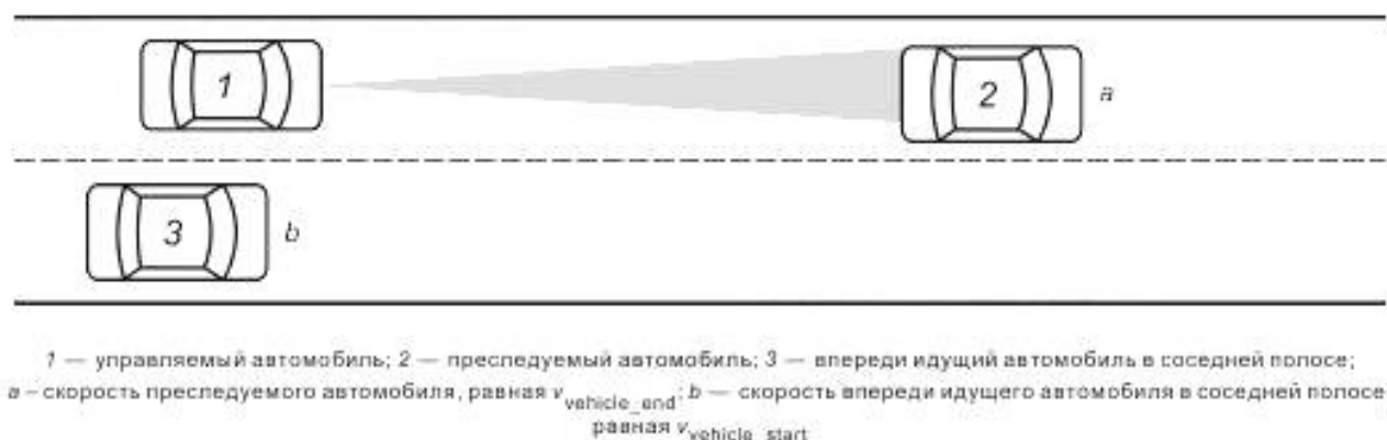
Рисунок 12 — Тестирование на выбор цели (конечные условия)
