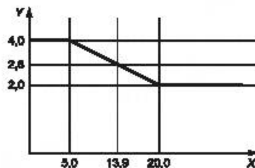
Рисунок 9 — Автоматическое ускорение
