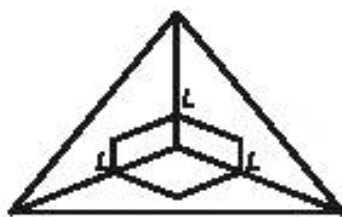
Рисунок А.6 — Угловой отражатель
