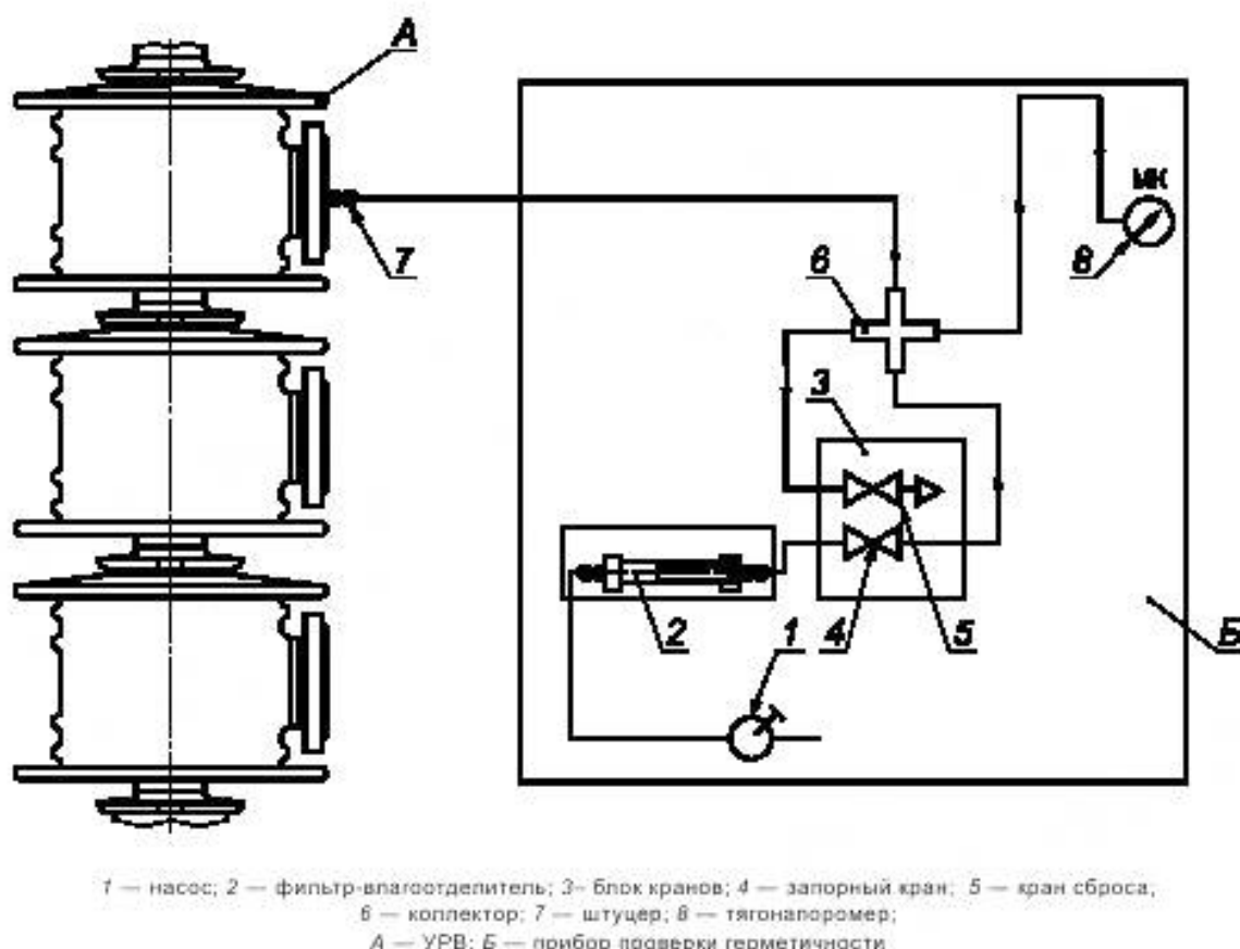
Рисунок 12.2 — Схема проверки герметичности УРВ
